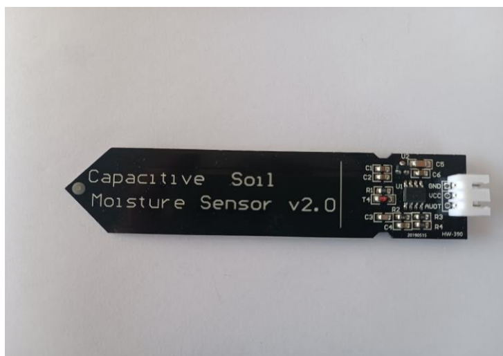
Obrázek 9 - Kapacitní senzor vlhkosti půdy
