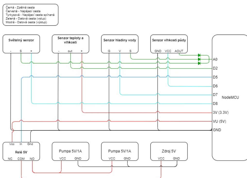
Obrázek 19 - Schéma zapojení
