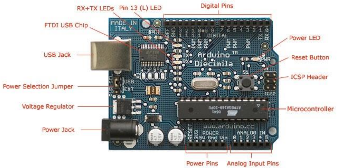
Obrázek 7 - Základová deska Arduino
