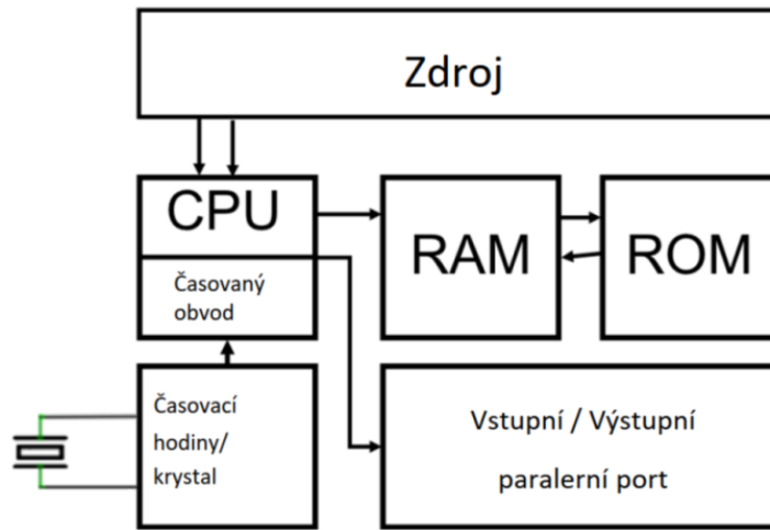
Obrázek 6 - Schéma mikrokontroléru
