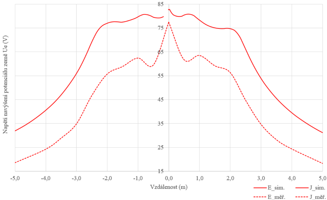
Graf simulace a měření rozložení potenciálu povrchu země v okolí zemních kruhů v přímce PO1 pro reálný numerický model, I_{RES} = 8,5 A
