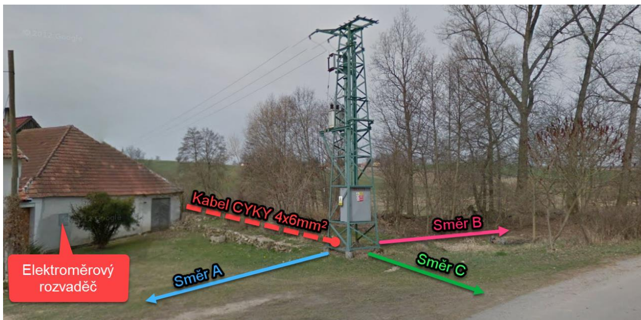
Obr. 9-2 Naznačené směry měření rozložení potenciálu země u DTS Kočí
