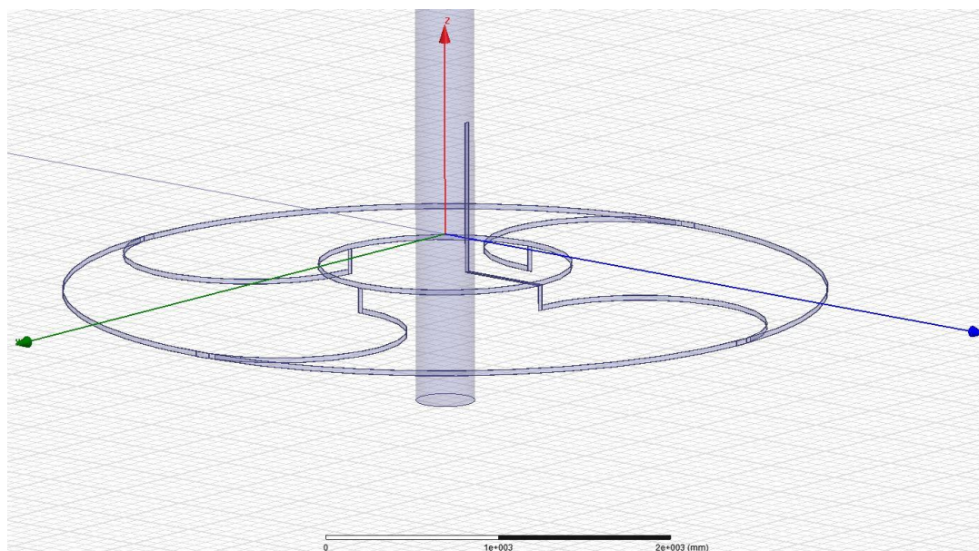
Obr. 8-3 Numerický model zemnicí soustavy v programu ANSYS Maxwell
