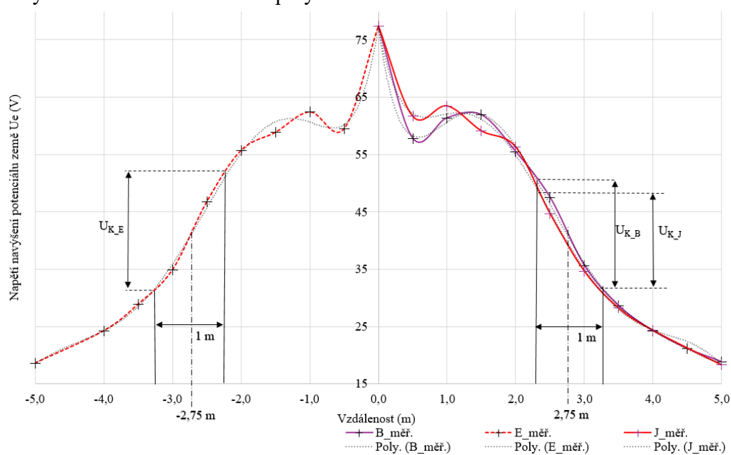
Obr. 9-19 Určení krokového napětí z grafu rozložení potenciálu země
