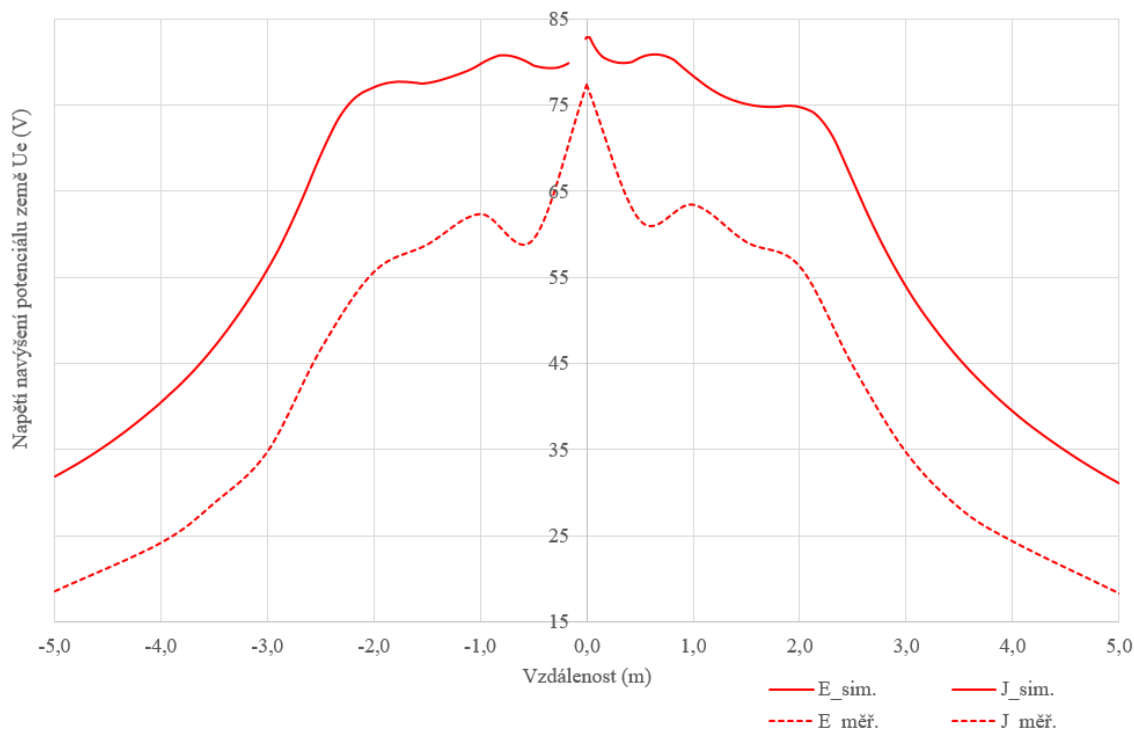
Obr. 9-15 Graf simulace a měření rozložení potenciálu povrchu země v okolí zemnicích kruhů v přímce POI pro reálný numerický model
