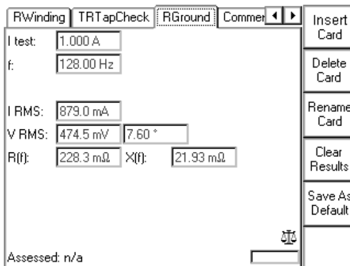
Obr. 3-7 Nastavení měřicího přístroje CPC 100 pro měření rezistivity půdy [9]
