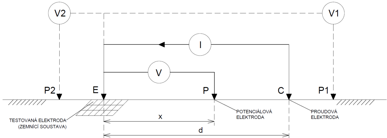
Obr. 4-1 Metoda potenciálového spádu [7]
