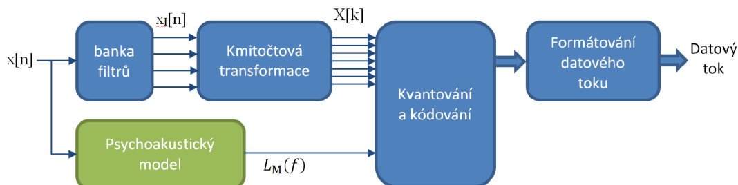
Obr. 1.1: Blokové schéma hybridního kodéru [2]
