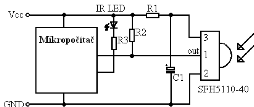
Obrázok 3.5: Jednoduchý senzor na detekciu prekážok
