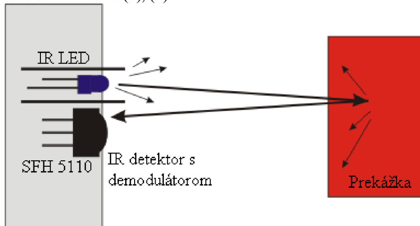
Obrázok 3.2: Princíp detekcie prekážky optoelektronickým sensorom
