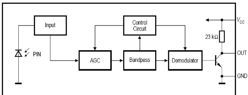
Obrázok 3.3: Bloková schéma obvodu SFH5110. Prevzaté z (7)
