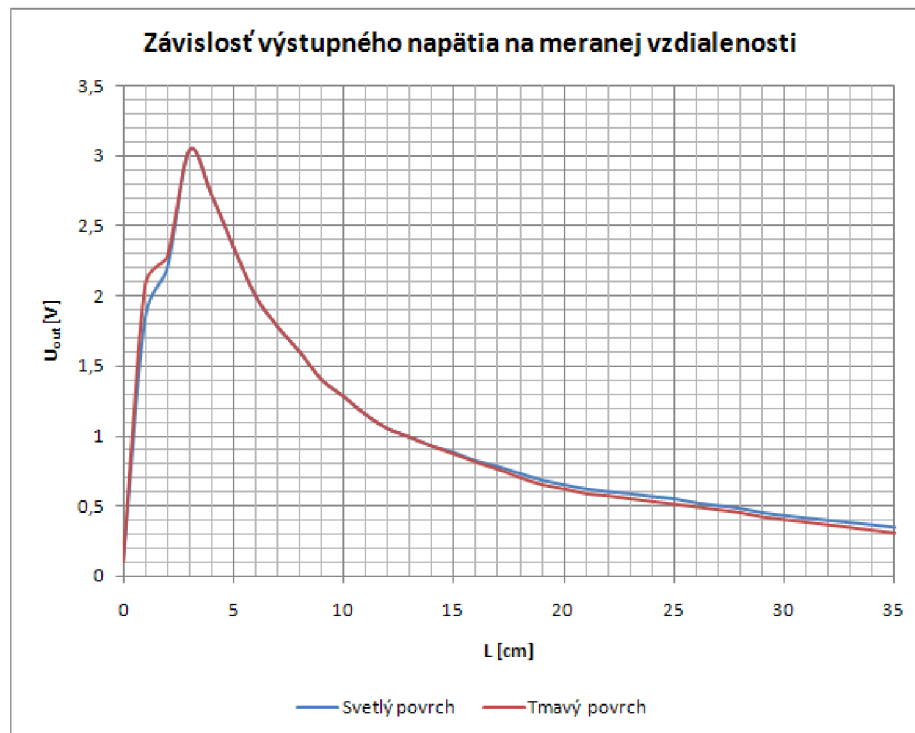
Obrázok 3.12: Nelineárny výstup senzoru GP2D120
