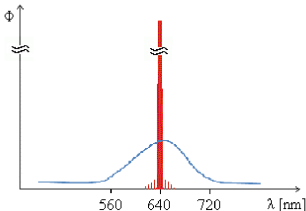
Obrázok 1.1: Spektrum laserovej diódy (červenou) a LED diódy (modrou)
