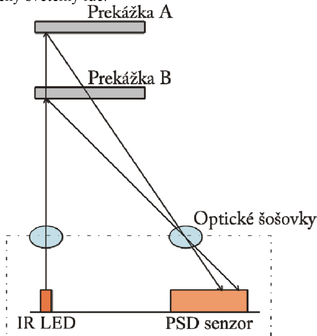
Obrázok 3.11: Meranie vzdialenosti pomocou triangulácie
