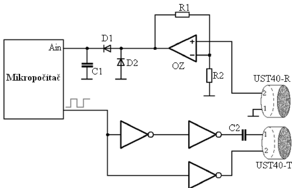
Obrázok 3.9: Příklad zapojenia ultrazvukového detektora prekážok
