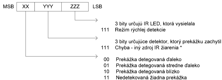
Obrázok 5.6: Formát odosielaných údajov - detekcia prekážky
