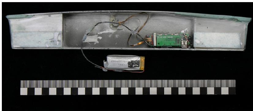
Obrázek 36: Falešný panel na bankomat s USB kamerou
