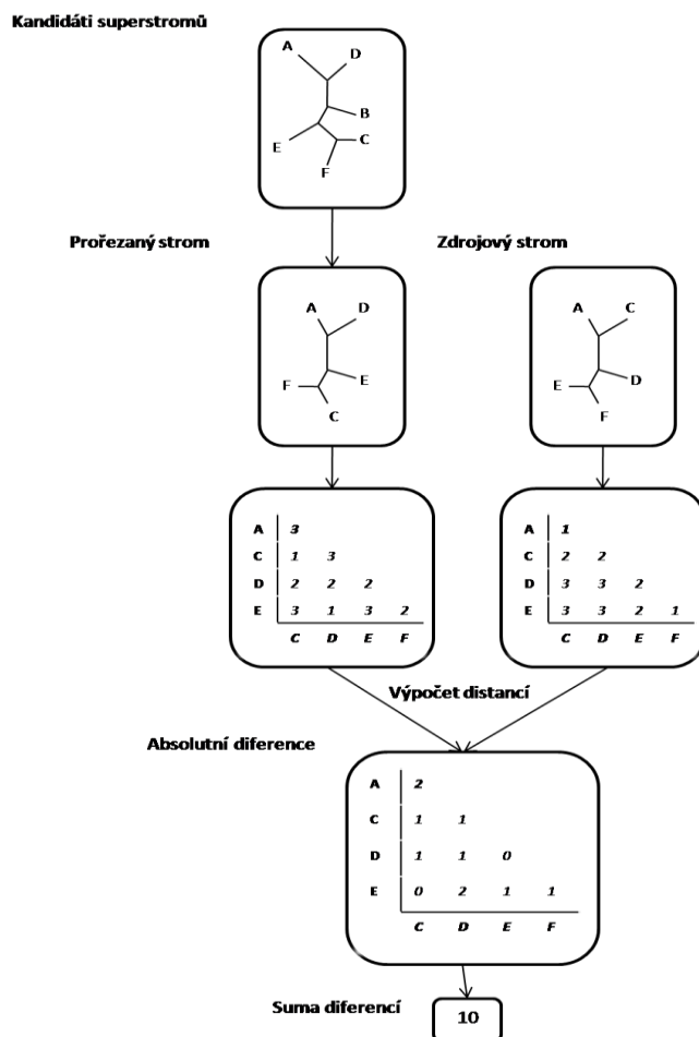
Obrázek 8: MSSA algoritmus [4]
