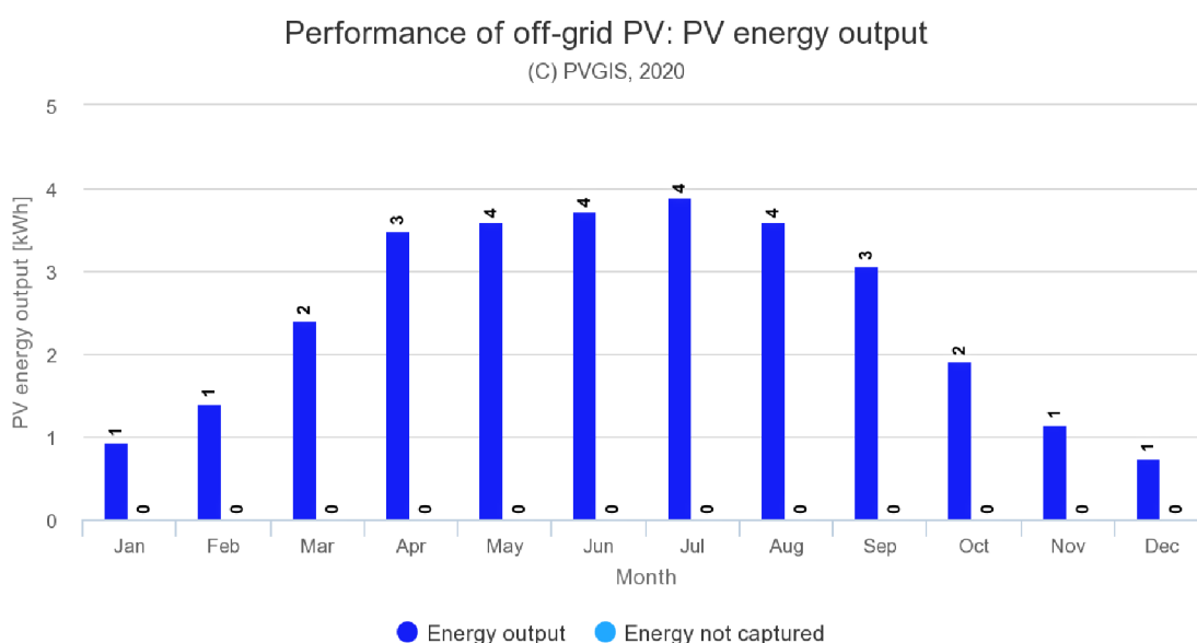
Obr. 4-8 Průměrná výroba elektrické energie FV panelu o výkonu 1 Wp [26]
