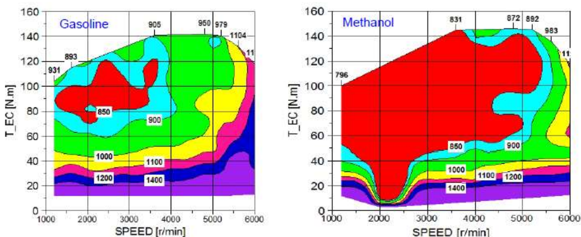
Graf 4 Porovnání produkce emisí \text{CO}_2 benzínového (vlevo) a metanolvého (vpravo) motoru [32]
