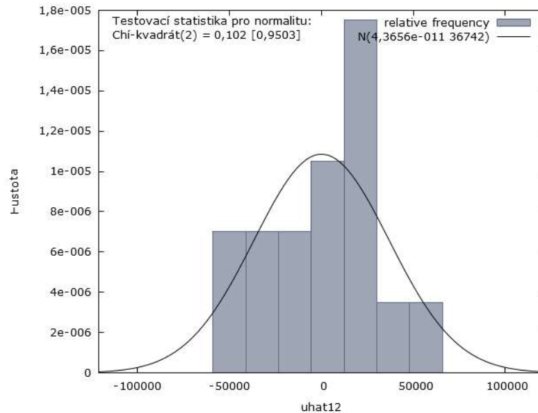
Obrázek 4: Graf normality reziduí první rovnice
