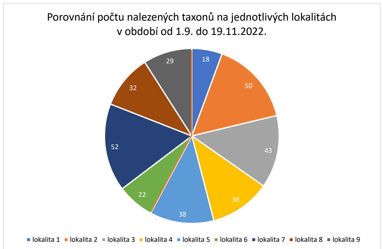
Graf 5: Porovnání počtu nalezených různých taxonů sinic a řas na jednotlivých lokalitách v období od 1.9. do 19.11.2022
