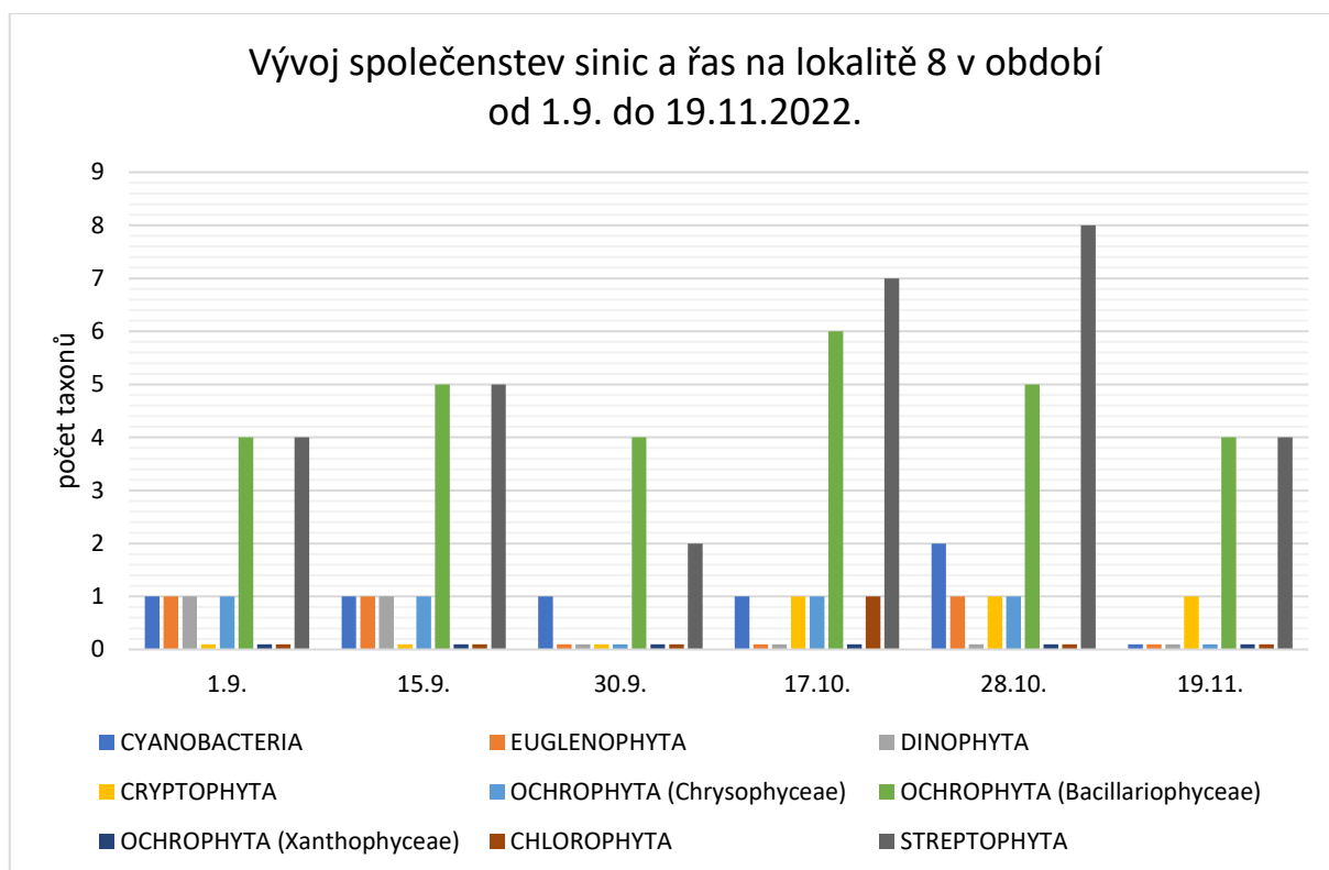
Graf 24: Vývoj společenstev sinic a řas na lokalitě 8 Velká tůň v období od 1.9. do 19.11.2022
