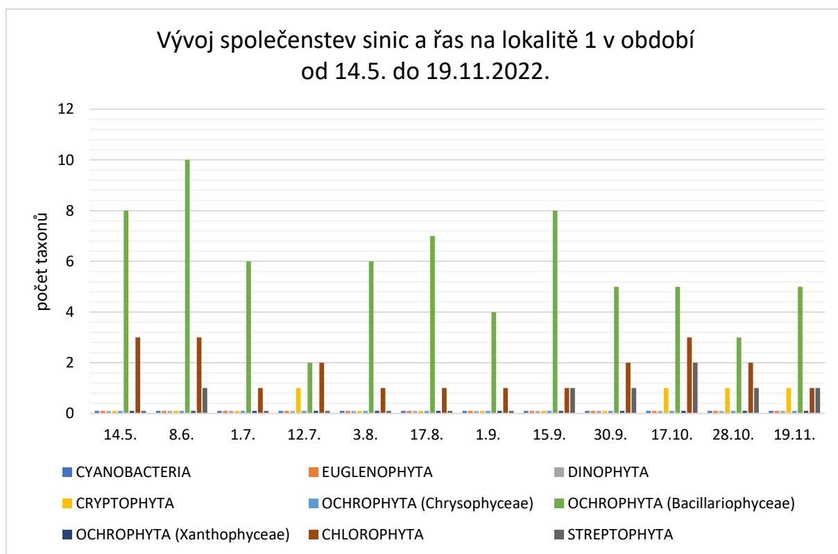
Graf 17: Vývoj společenstev sinic a řas na lokalitě 1 Lesní tůň v období od 14.5. do 19.11.2022
