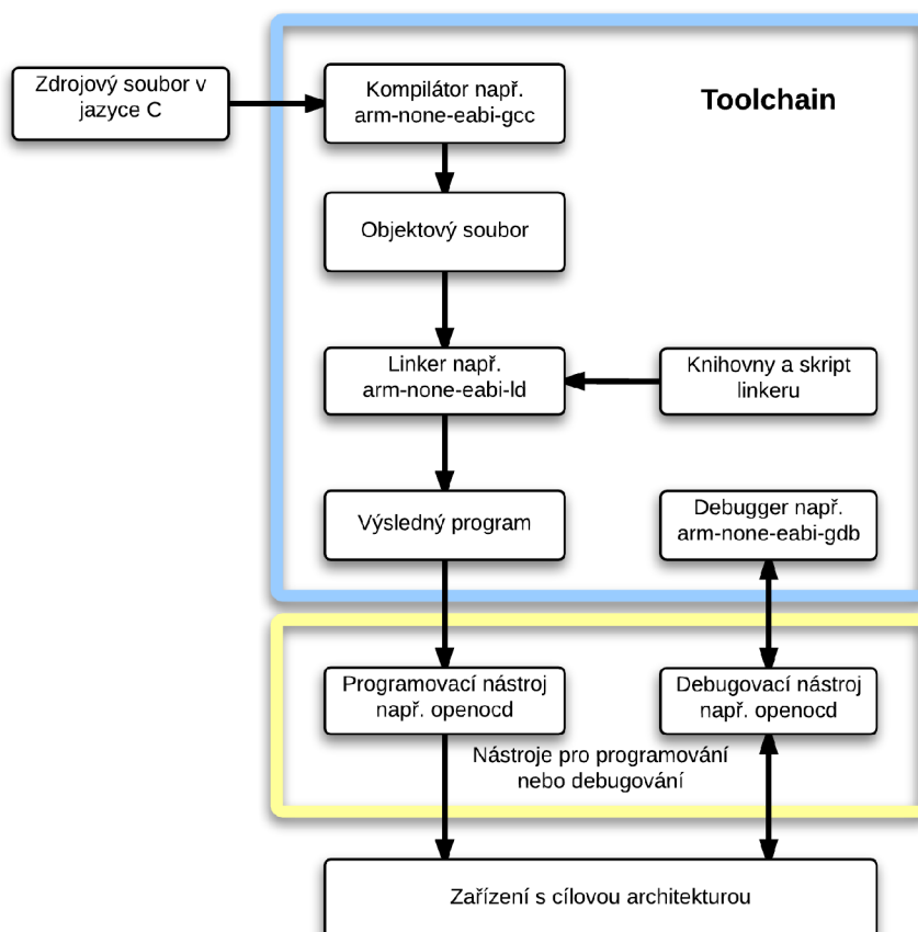
Obrázek 2.1: Struktura toolchainu [14]
