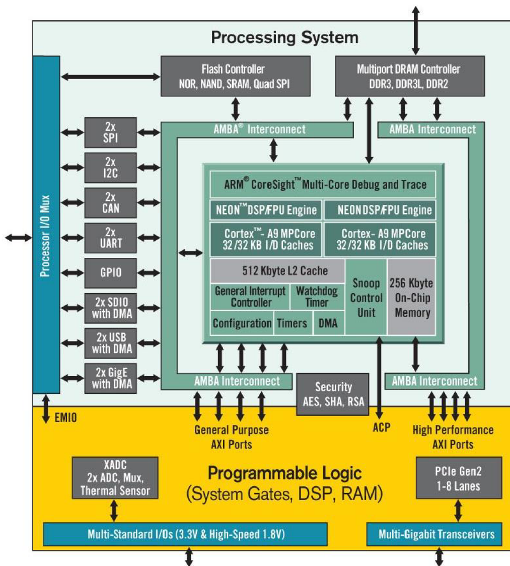
Obrázek 2.2: Diagram procesorového systému Zynq-7000 [15]
