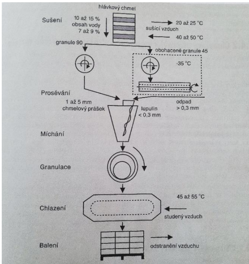
Obrázek 4 - schéma přípravy pelet 90 a 45 [2]
