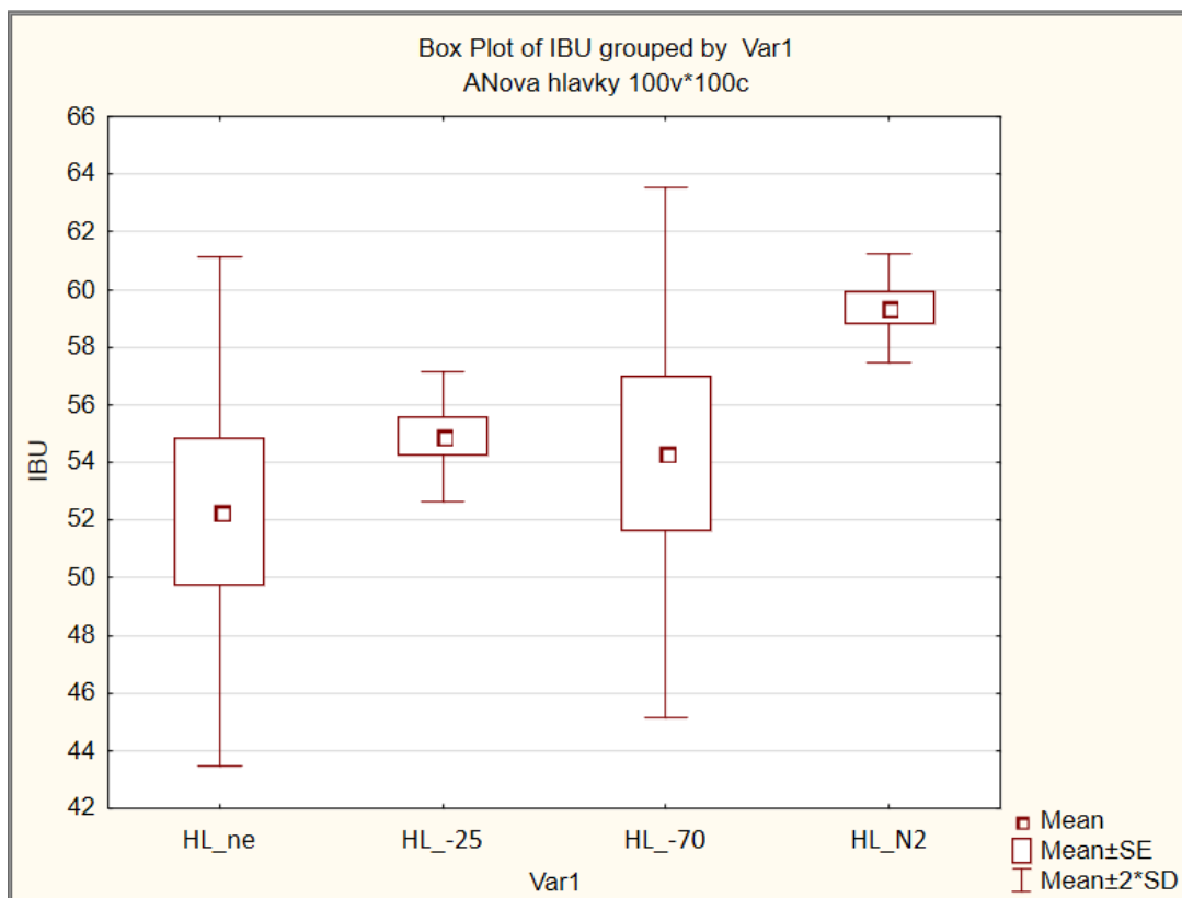
Obrázek 13 - boxový graf znázorňující statistické rozdíly mezi hořkostí pro jednotlivé úpravy lisovaných chmelových hlávek
