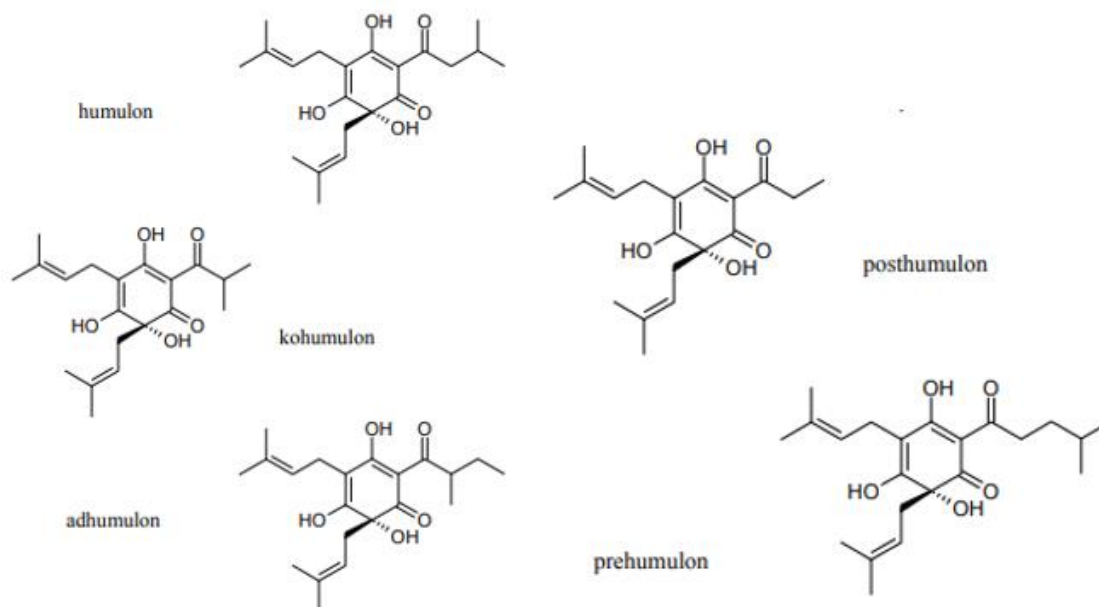
Obrázek 2 - strukturní vzorce \alpha -hořkých kyselin [3]
