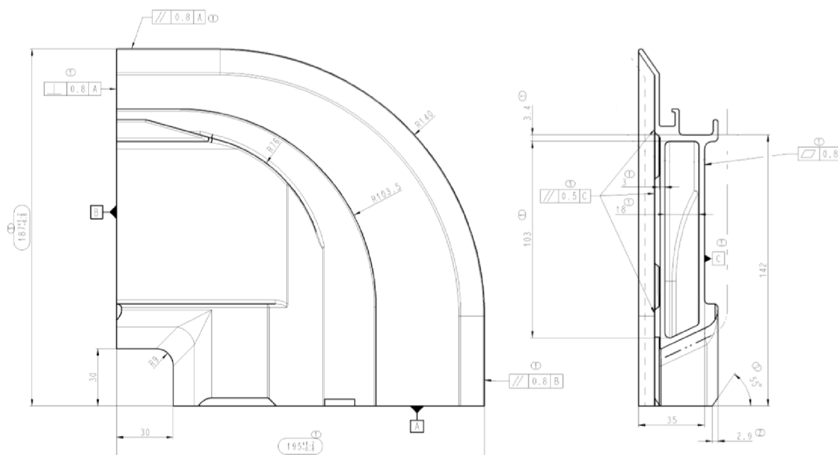
Obr. 6 Rozměry součásti
