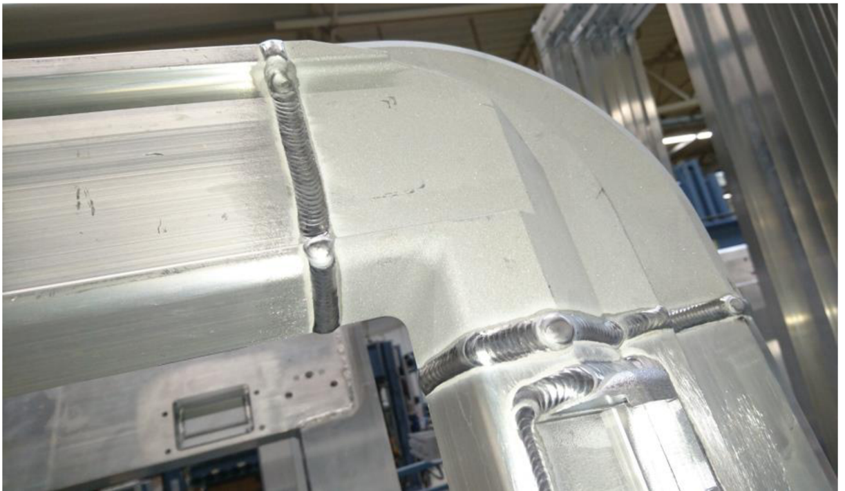
Obr. 8 Rám po navaření
