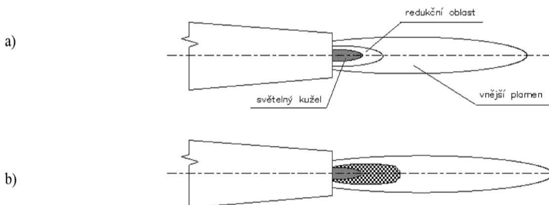
Obr. 16 Neutrální a redukční plamen [19]
