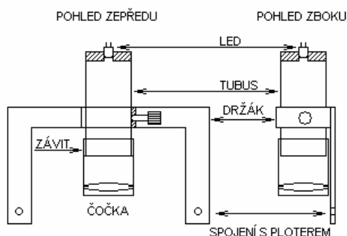
Obr. 11 Optický systém pro LED diody
