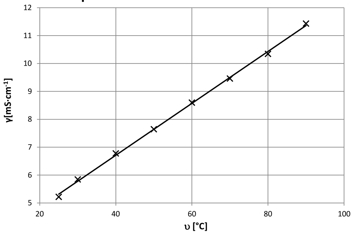
Obr. 28: Teplotní závislost vzorku SI 50 % + DMC 50 % + LiClO 4
