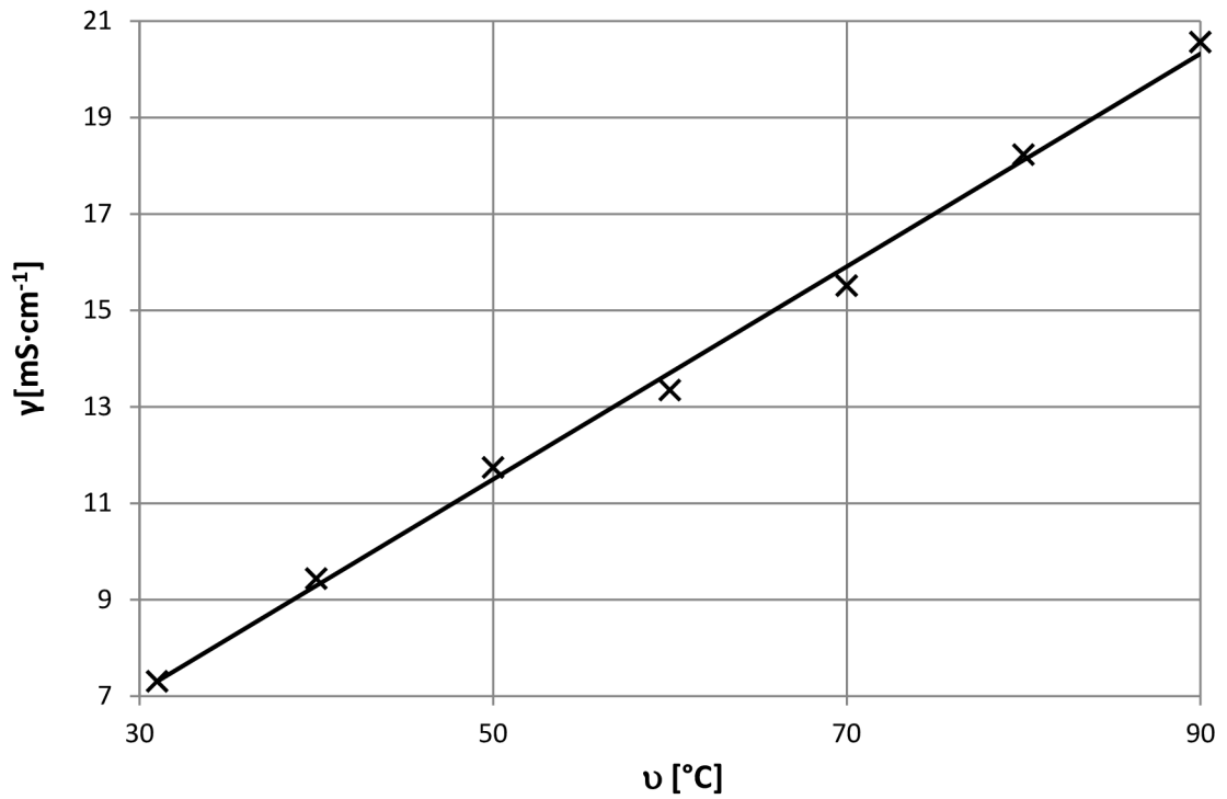
Obr. 31: Teplotní závislost vzorku SI 50 % + DMSO 50 % + LiClO 4
