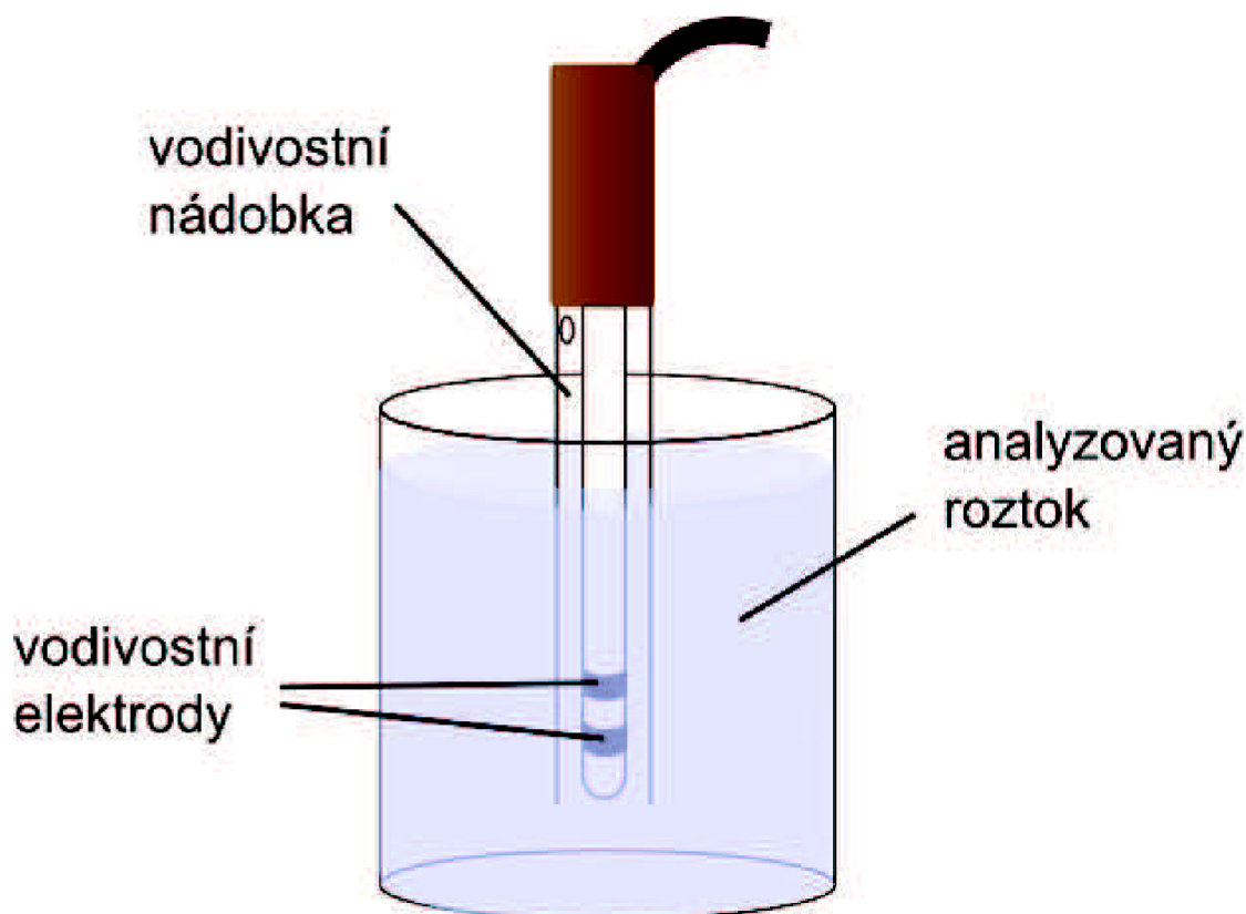
Obr. 2: Konstrukčního uspořádání ponorné nádoby[5]
