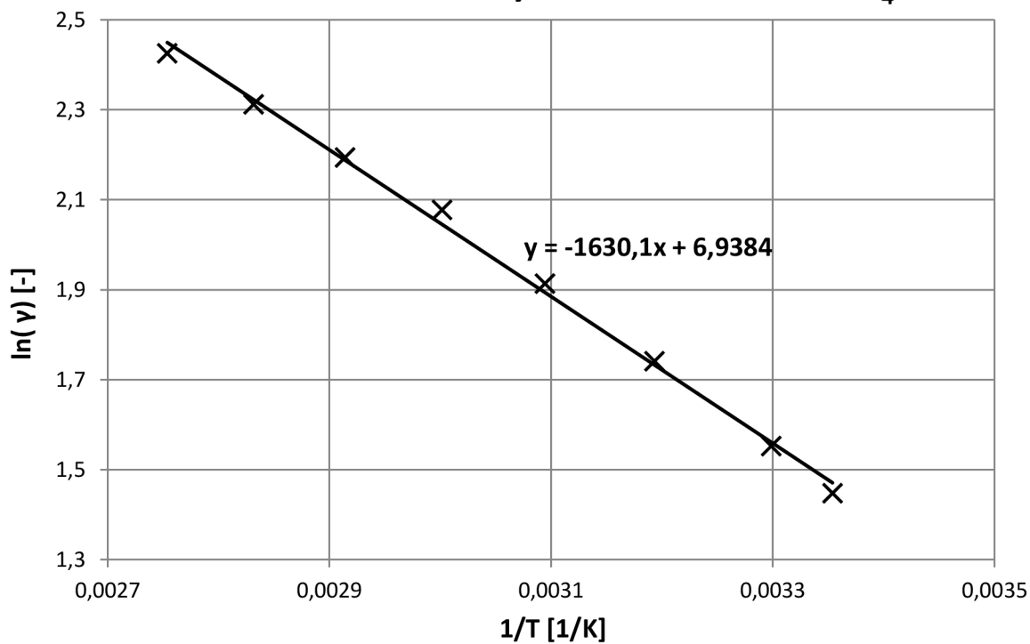
Obr. 49: Graf závislosti \ln(\gamma) na \frac{1}{T} vzorku Sl 80 % + DMC 20 % + LiClO 4
