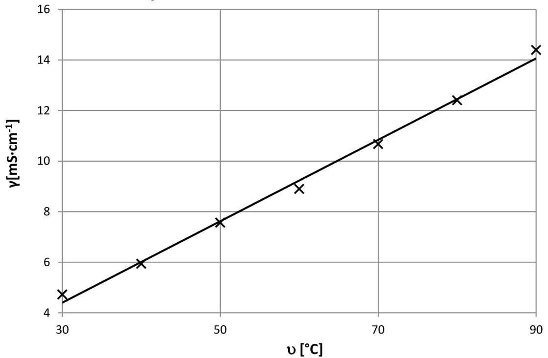
Obr. 32: Teplotní závislost vzorku SI 80 % + DMSO 20 % + LiClO 4
