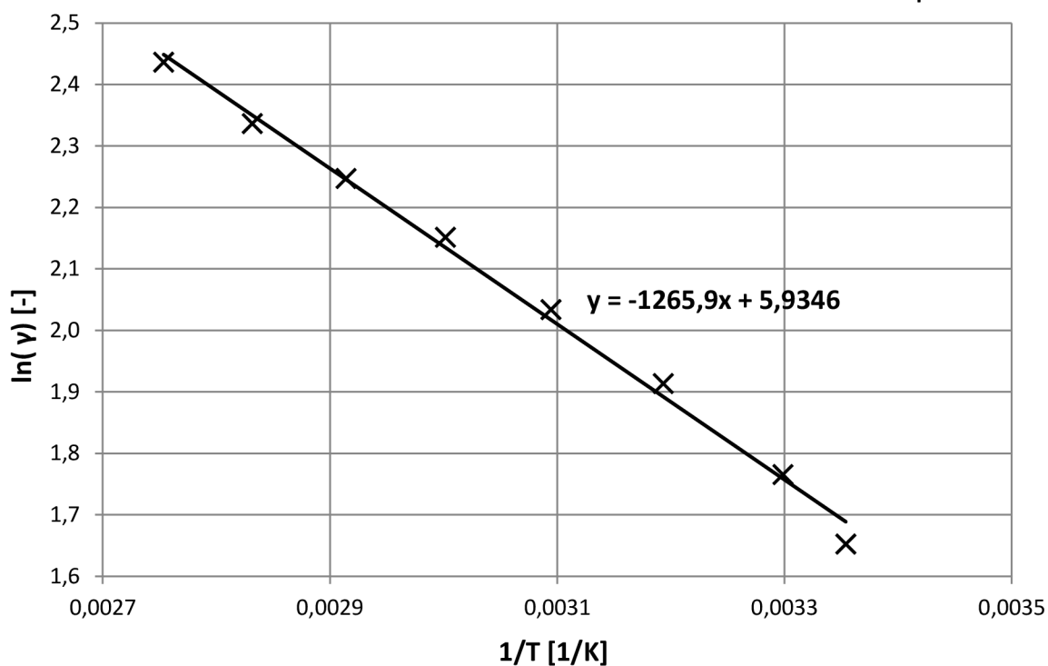
Obr. 48: Graf závislosti \ln(\gamma) na \frac{1}{T} vzorku Sl 50 % + DMC 50 % + LiClO 4
