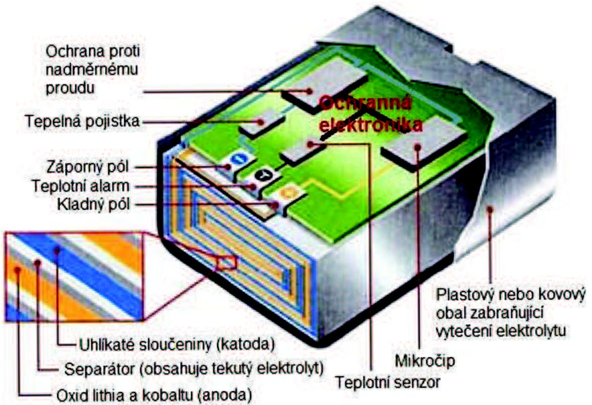
Obr. 1: Řez Li-ion článkem [3]
