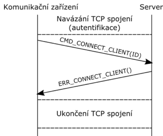
Obr. 5.3: Princip zahájení a ukončení spojení pomocí D4 zpráv mezi serverem a komunikačním zařízením
