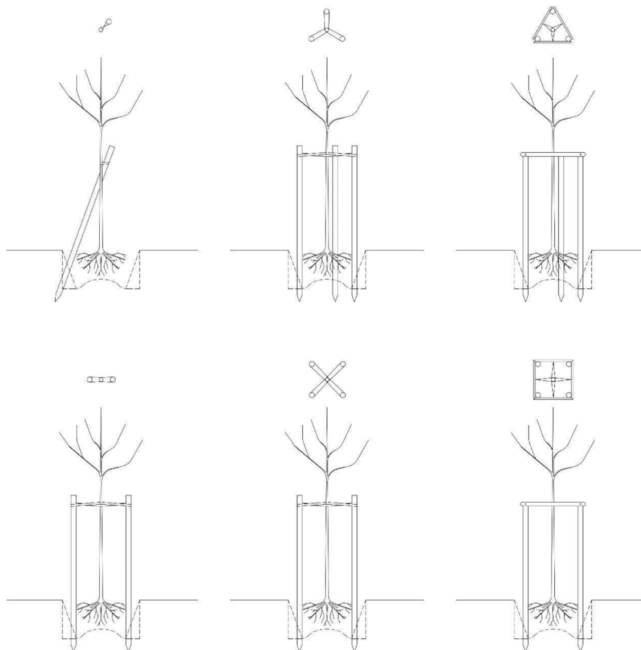
Obrázek 10 – Typy nadzemního kotvení (Kolařík et al., 2021).
