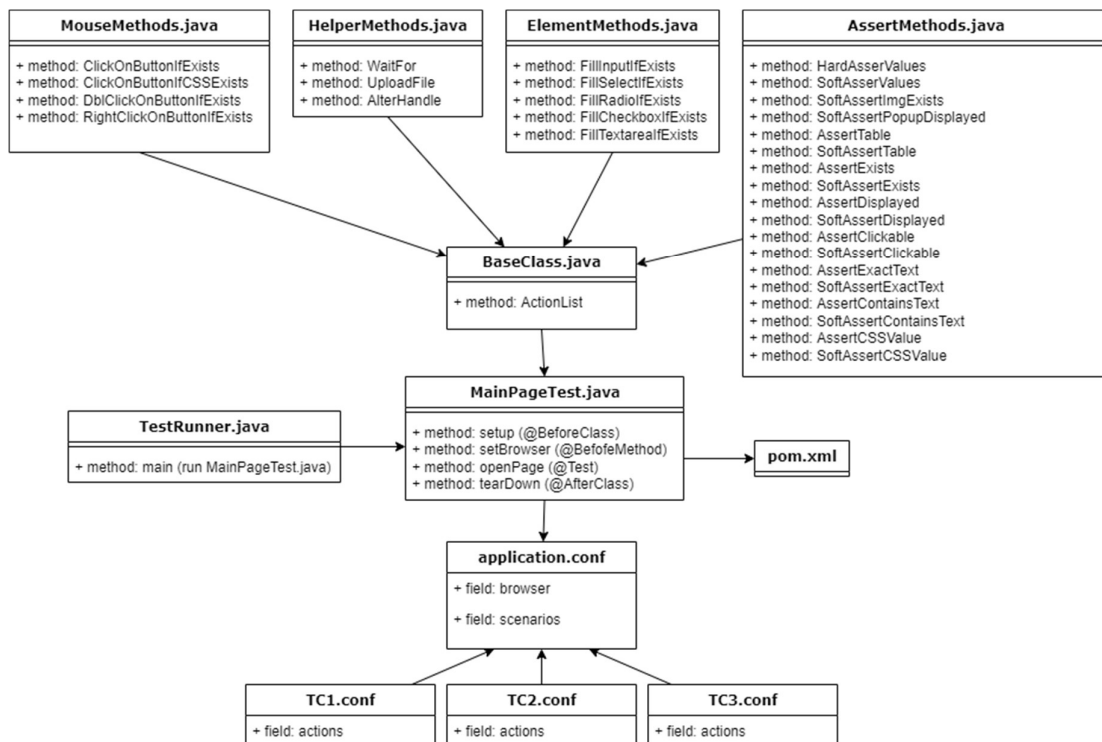
Obrázek 19 – Class diagram překladače
