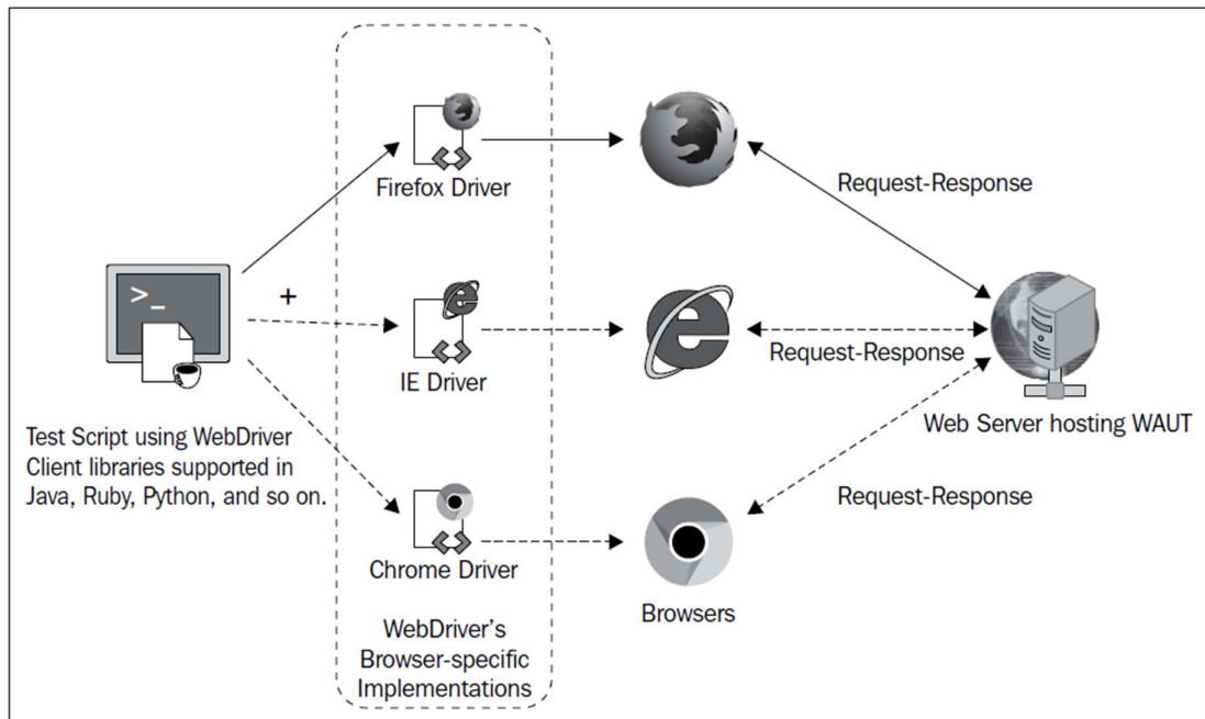
Obrázek 11 – Princip fungování Selenium WebDriver [13]
