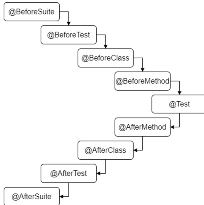
Obrázek 14 – Hierarchie anotací TestNG
