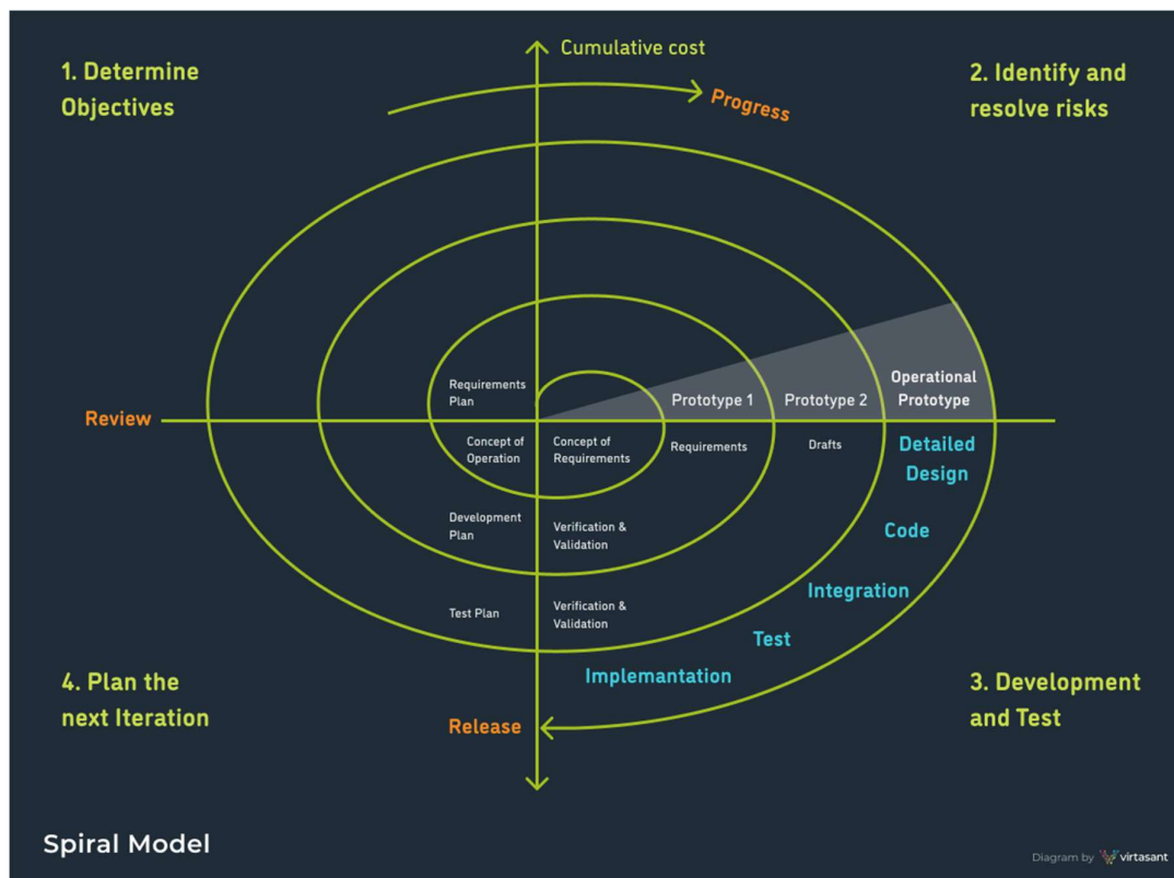
Obrázek 7 – Spirálový model [4]
