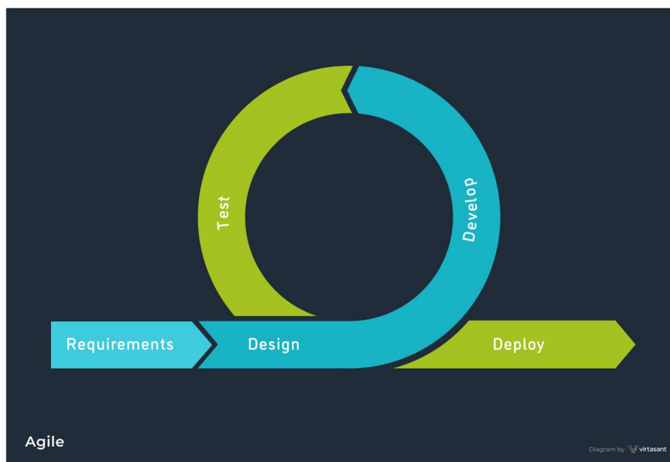
Obrázek 9 – Agilní model [4]
