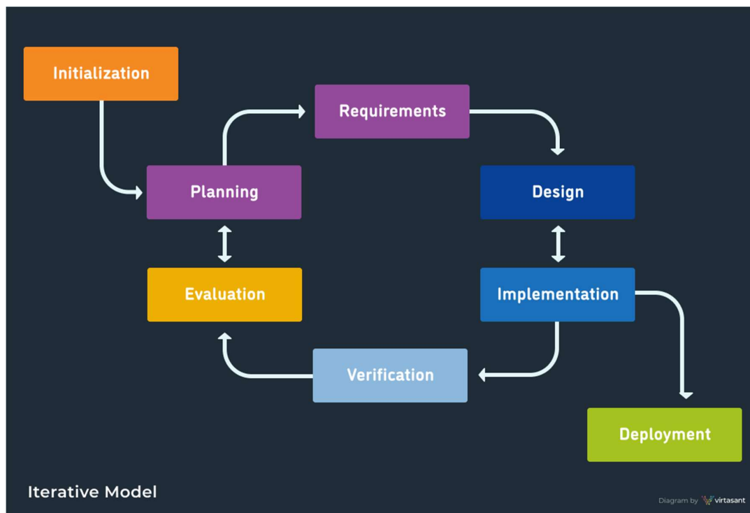
Obrázek 6 – Iterativní model [4]
