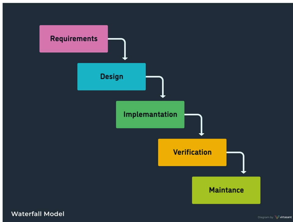
Obrázek 4 – Waterfall Model [4]
