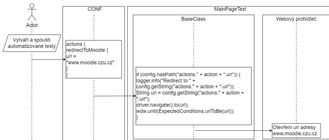
Obrázek 18 – Sekvenční diagram
