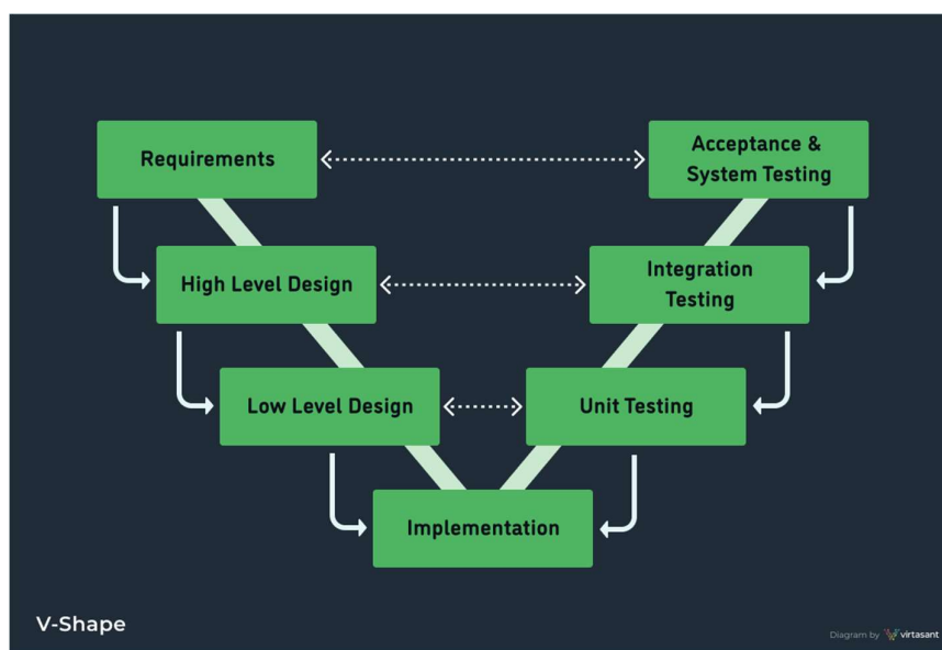
Obrázek 8 – V-model [4]
