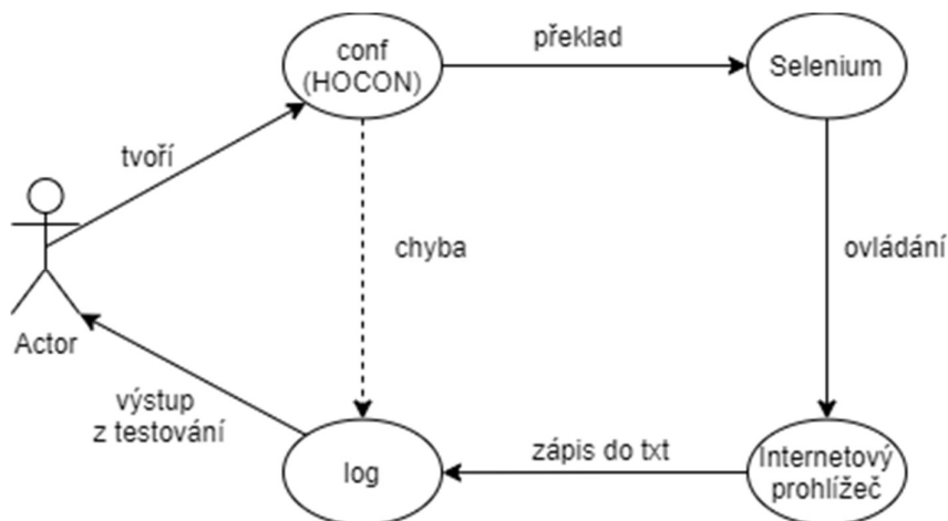
Obrázek 16 – Návrh překladače
