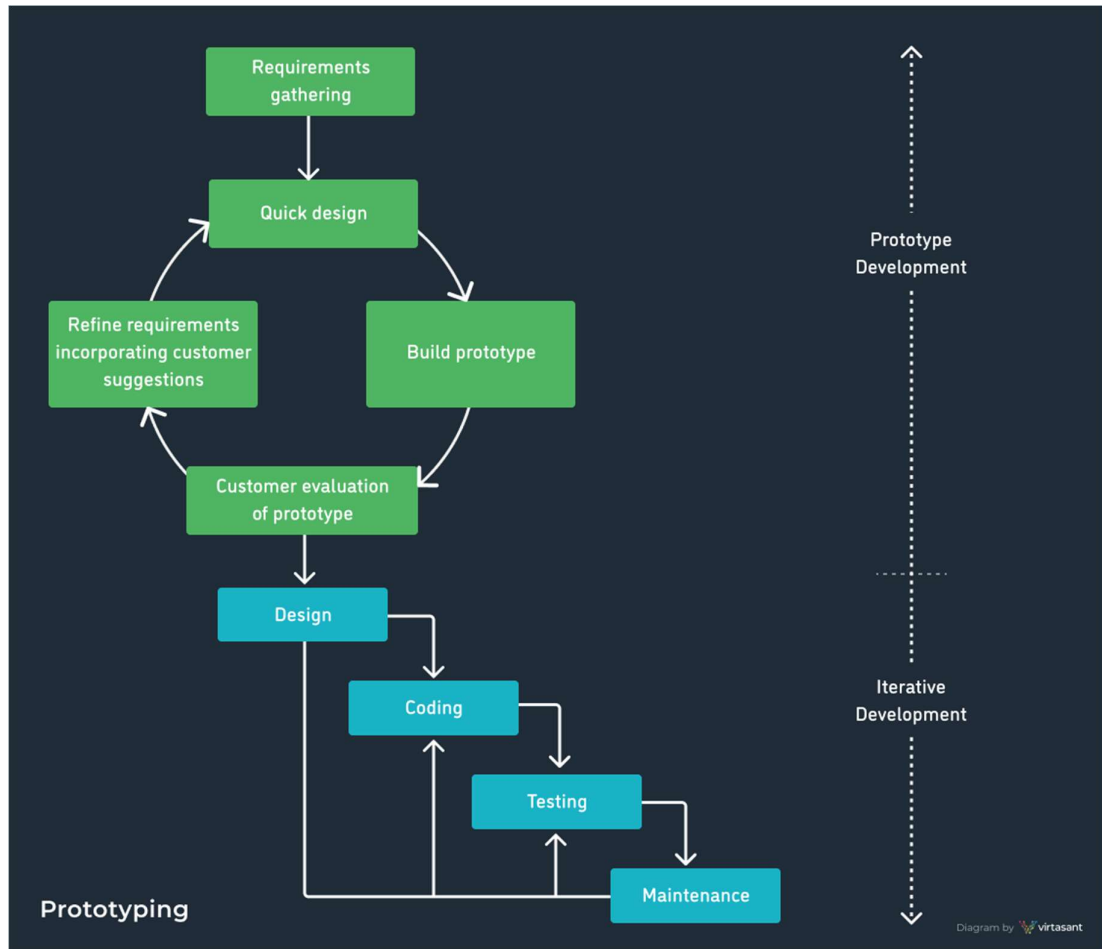
Obrázek 5 – Prototypování [4]
