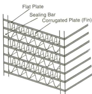
Obr. 2.10 Základní konstrukce lamelového tepelného výměníku. Obrázek také ukazuje uspořádání pro souprůd, protiprůd a křížící se proudy.
