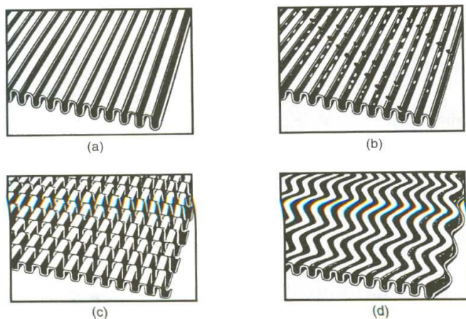
Obr. 2.11 Typy žebor v lamelových tepelných výměnících
