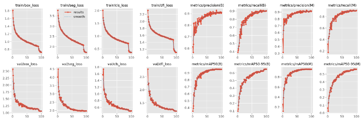
Obrázek 36 – YOLO průběh učení, LR 0.01, 100 epoch
