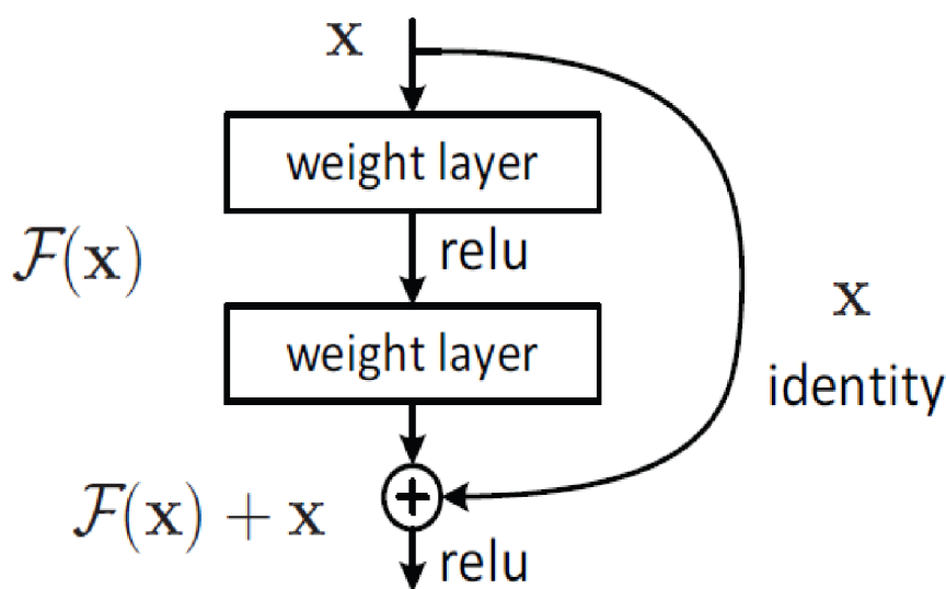
Obrázek 16 – Reziduální propojení [6]
