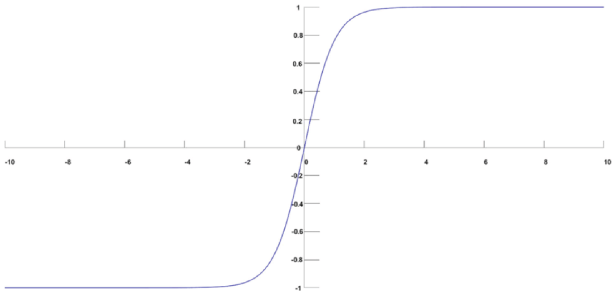
Obrázek 9 - Softmax funkce [30]
