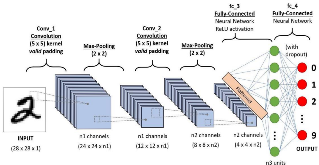
Obrázek 15 – CNN architektura [36]
