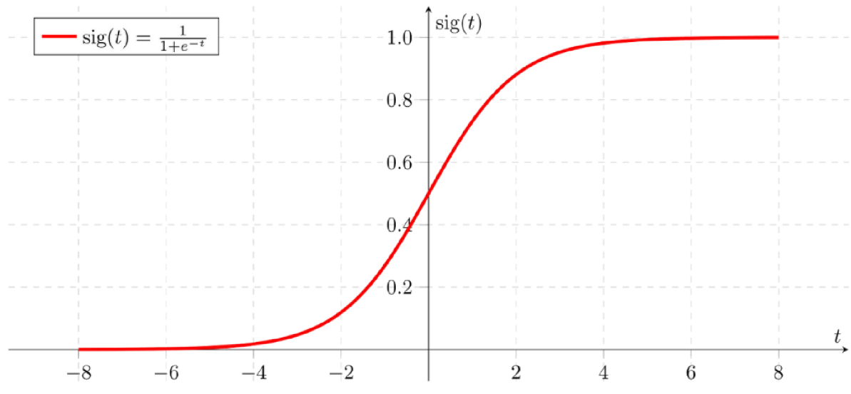
Obrázek 11 – Sigmoida funkce [32]
