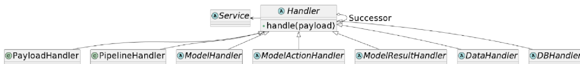
Obrázek 30 – UML class diagram, handler vrstva
