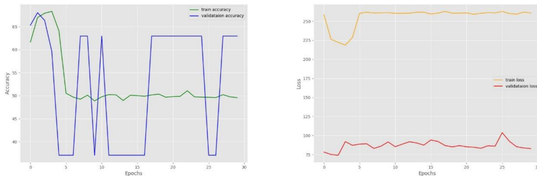
Obrázek 46– CNN průběh učení hranové obrazy, LR 0.01, 30 epoch
