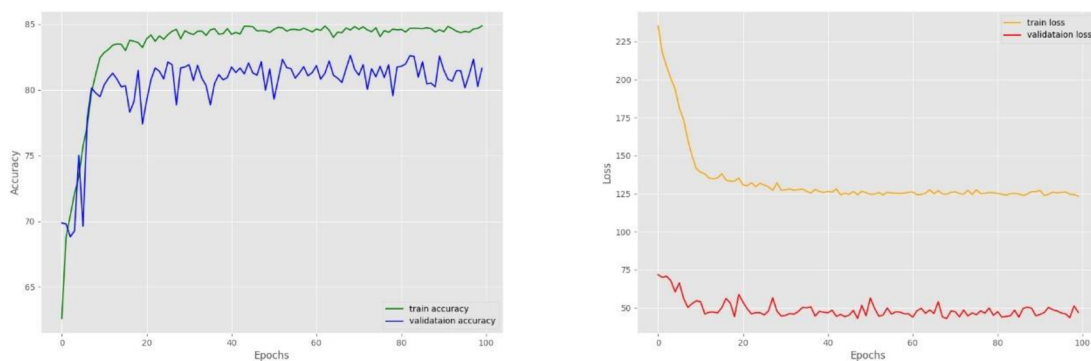
Obrázek 47– CNN průběh učení barevné obrazy, LR 0.01, 100 epoch
