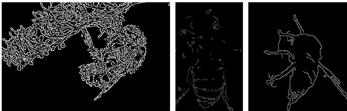
Obrázek 21 – Edge obraz 18
