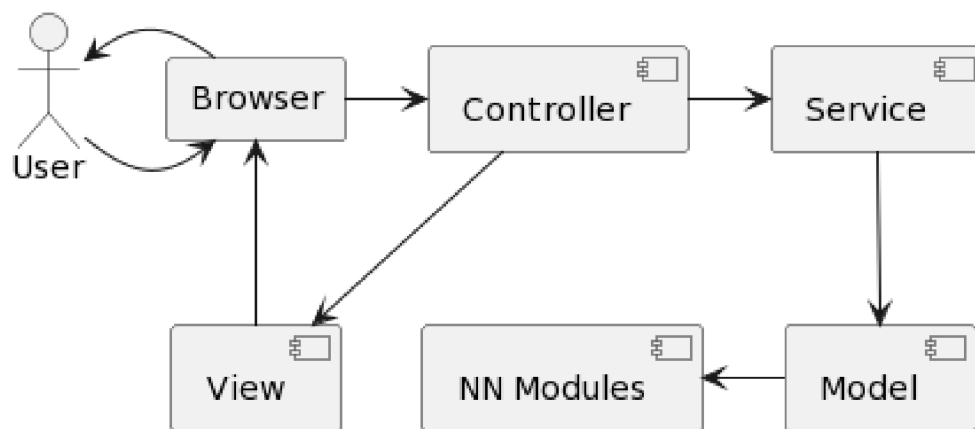
Obrázek 27 – Architektura aplikace
