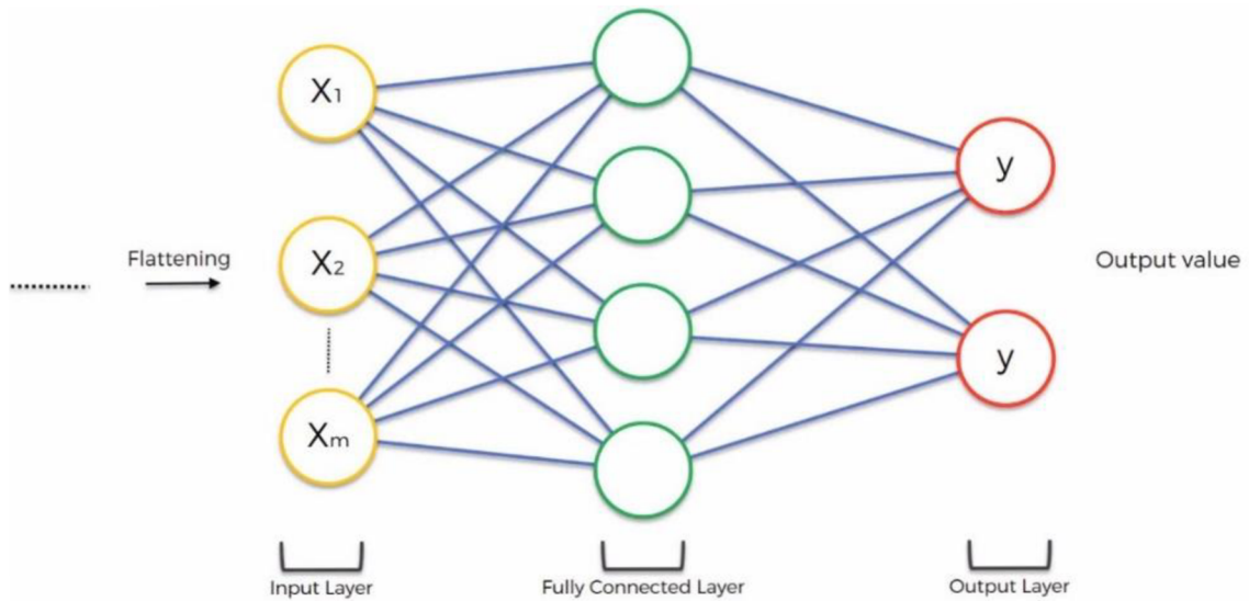
Obrázek 14 – FC vrstva [35]
