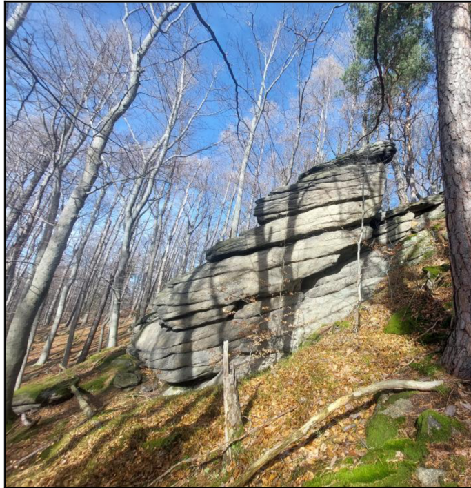
Obr. 33. Jedno ze žulových skalisek na Borovém vrchu s dobře patrnými exfoliačními deskami (foto: Malíková, 2024)
