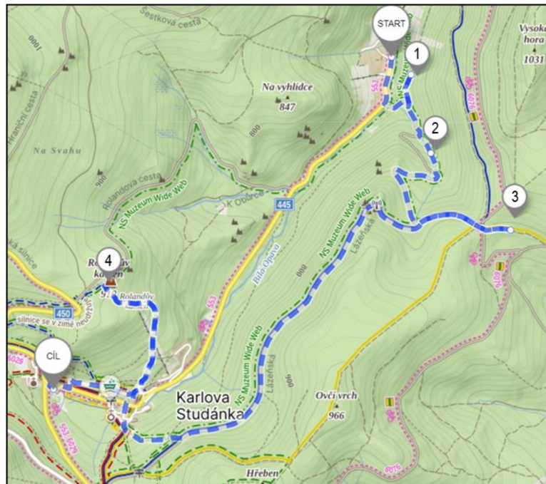
Obr. 6. Trasa exkurze Ludvíkov – Karlova Studánka (start- aut. zast. Stonožka, 1. odvaly rud, 2. ložisko Ludvíkov, 3. ložisko Hláska, 4. Rolandův kámen, cíl-geologická exkurze) (zdroj: www.mapy.cz , 2024)
