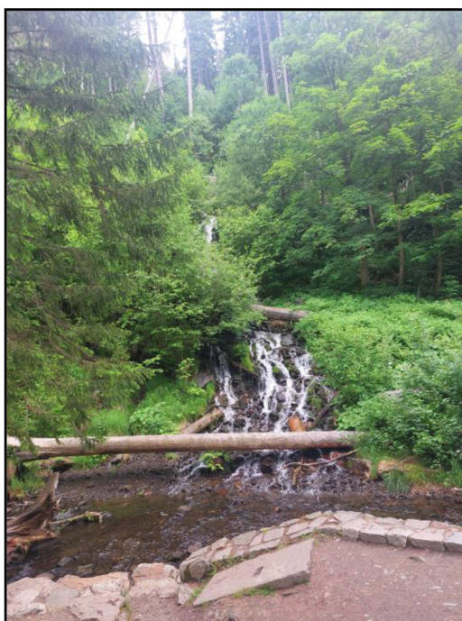
Obr. 16. Uměle vytvořený vodopád v Karlově Studánce (foto: Malíková, 2023)
