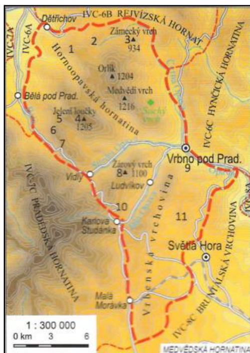
Obr. 4. Medvědká hornatina (Bína a Demek, 2012) Obr. 5. Pradědská hornatina (Bína a Demek, 2012)
