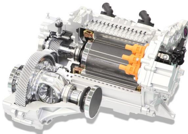
Obr. 2.3 Hnacie ústrojenstvo – Volkswagen e-Golf [24]
