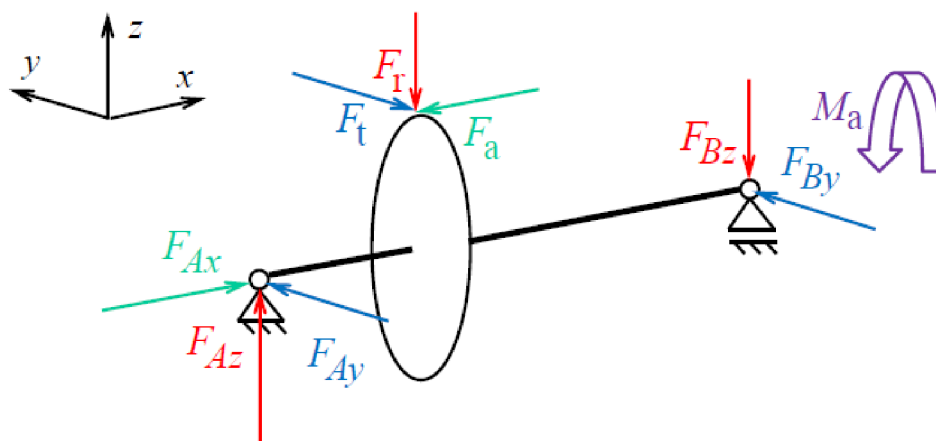
Obr. 5.2 Zatiaženie hriadeľa „a“
