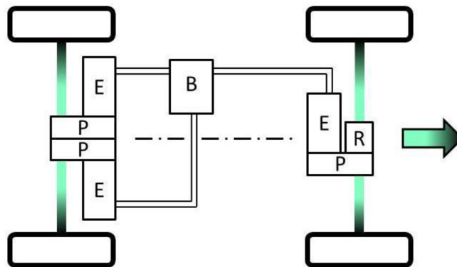
Obr. 1.2 Pohón tromi elektromotormi [2]
