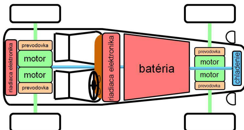
Obr. 3.3 Schéma pohomu
