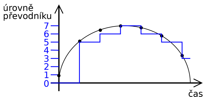
Obrázek 2.14: Činnost 3-bitového AD převodníku. Černá čára znázorňuje spojité signál, který je výstupem ze senzoru. Černé puntíky označují vzorky odebrané vzorkovačem. Modrou čarou je vyznačen průběh digitalizovaného signálu.
