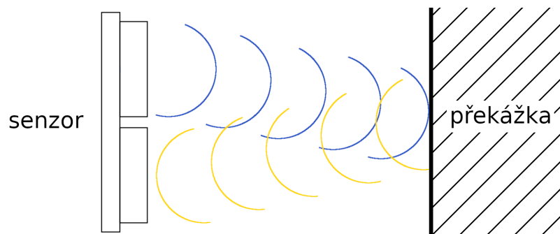
Obrázek 2.5: Princip měření vzdálenosti ultrazvukovým senzorem. Vysílač mění přivedenou elektrickou energii na mechanické vlnění. Na senzor působí odražené vlny, a ten mění mechanickou energii zpět na elektrickou.
