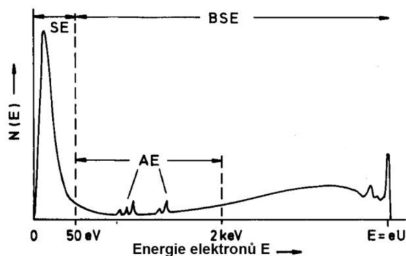
Obr. 2.3 Spektrum emitovaných elektronů [8]
