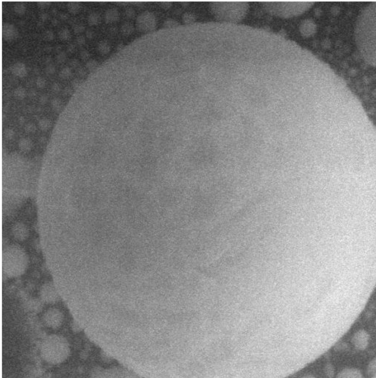
Obr. 6.15 Snímek kuličky cínu, p = 900 \text{ Pa} , nast.2, F:62.5/18.1, ( A1 = 0,6 \text{ mm} ), zv. 15000x
