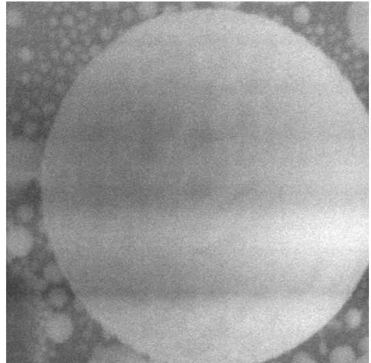
Obr. 6.16 Snímek kuličky cínu, p = 1000 \text{ Pa} , nast.2, F:57.1/16.0, ( A1 = 0,6 \text{ mm} ), zv. 15000x
