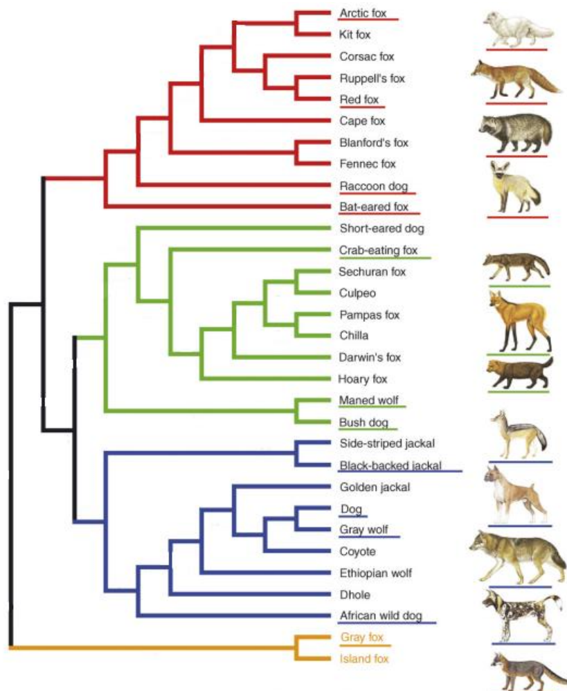
Obrázek 4. Molekulární fylogeneze čeledi Caninae – Červená větev značí skupinu lišky (Vulpini), zelená větev jihoamerické psovitě šelmy (Cerdocyonina), modrá větev značí druhy podobné vlka obecnému, žlutá skupina značí lišky šedé a ostrovní. Podtržené názvy jsou doplněny ilustracemi (Wayne & Ostrander 2007).
