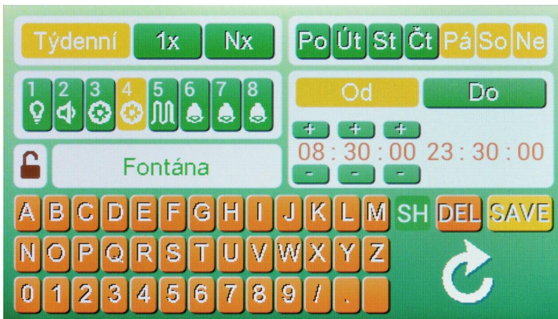
Obr. 19 Příklad použití ovladače (widgety tlačítek a klávesnice)
