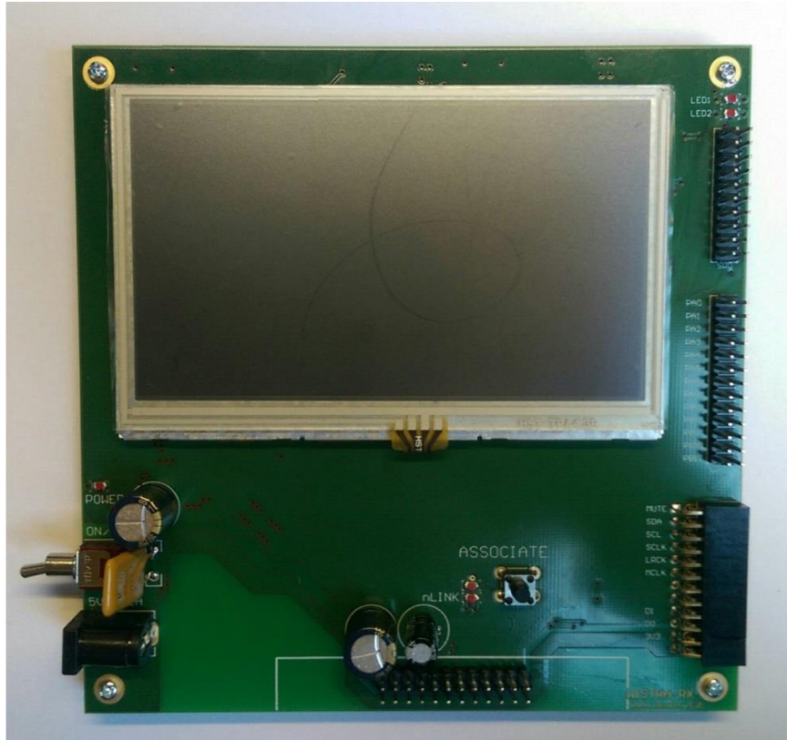
Obr. 13 Hotová vývojová deska přijímače - pohled shora
