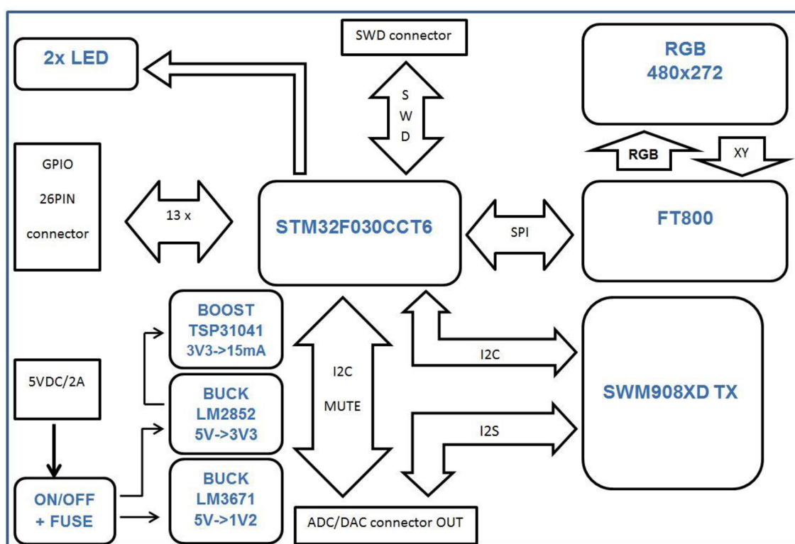
Obr. 4 Blokové schéma vývojové desky vysílače
