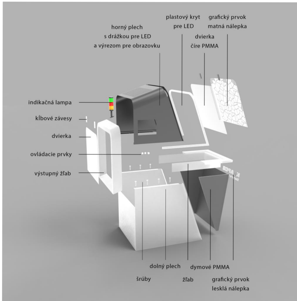
Obr. 6-4 Vonkajšie komponenty
