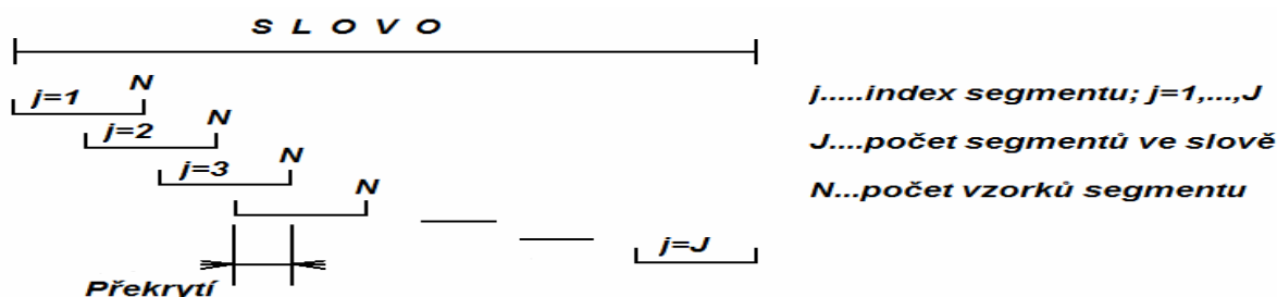
Obr. 3.3 Princip segmentace
