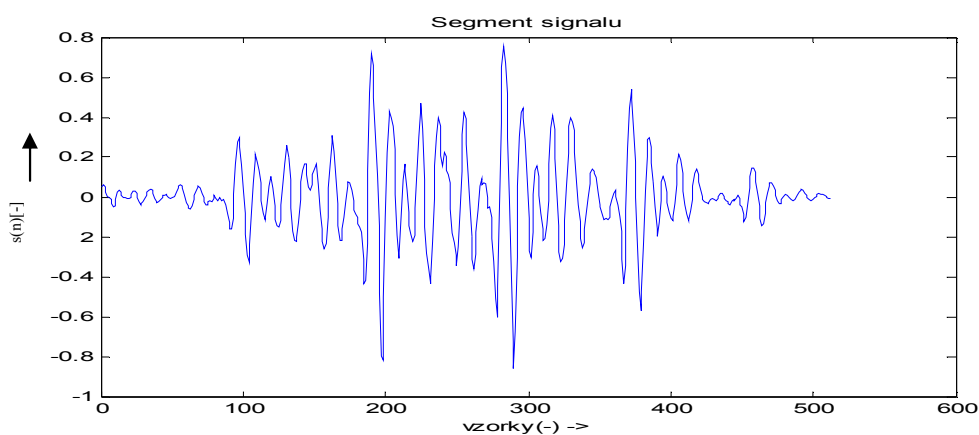
Obr. 3.5 Jeden segment signálu váhovaný Hammingovým oknem
