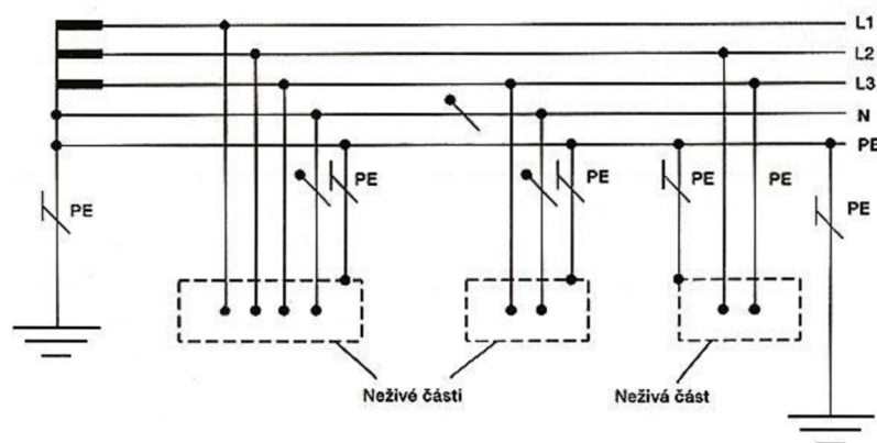
Obrázek 4: Síť TN-S [3]
