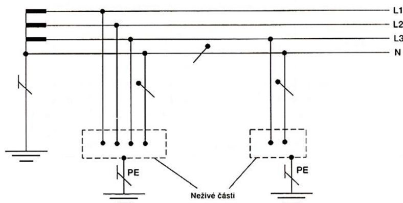
Obrázek 2: Síť TT [3]
