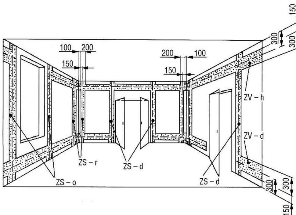
Obrázek 8: Instalační zóny [5]
