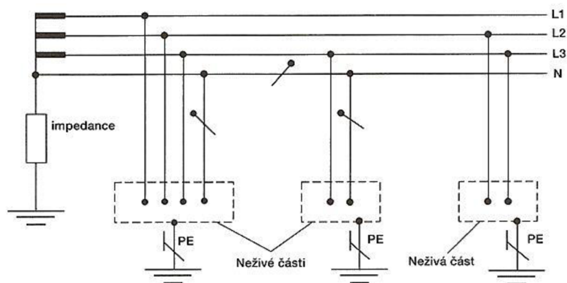
Obrázek 1: Síť IT [3]
