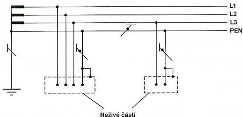
Obrázek 3: Síť TN-C [3]
