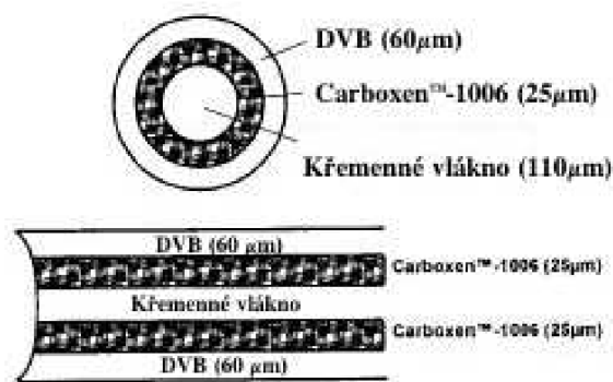
Obr. 2.12: Schema kombi. SPME vlákna DVB-PDMS přes vrstvu CAR TM -PDMS
