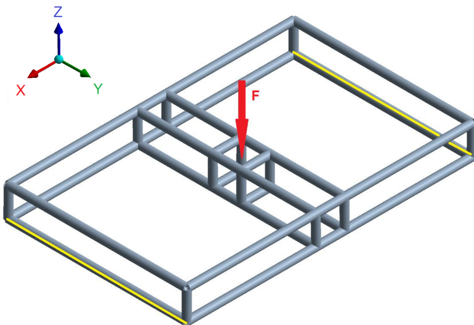
Obrázek 5:1 Okrajové podmínky pro výpočet
