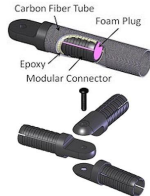
Obrázek 3:5 Spojka DragonPlate [3]
