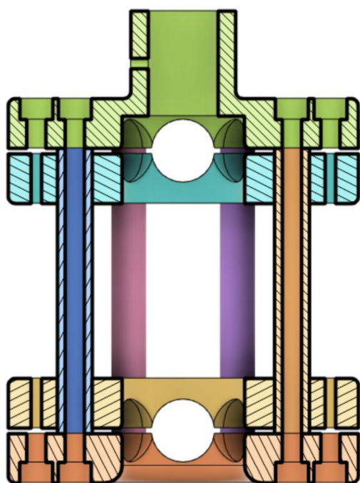
Obrázek 5:14 Řez středovým unašečem [7]
