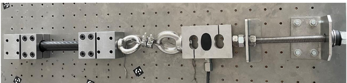
Obrázek 5:10 Finální sestava užitá pro provedení zkoušky tahem
