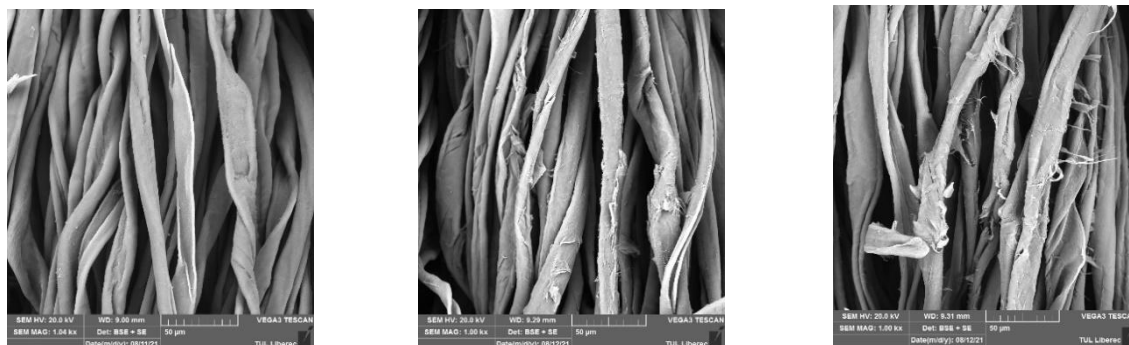
Obrázek 41 vlákna trička Calvin Klein A před praním a po padesáti cyklech praní v pracím prostředku Woolite Darks denim Black a Persil Color
