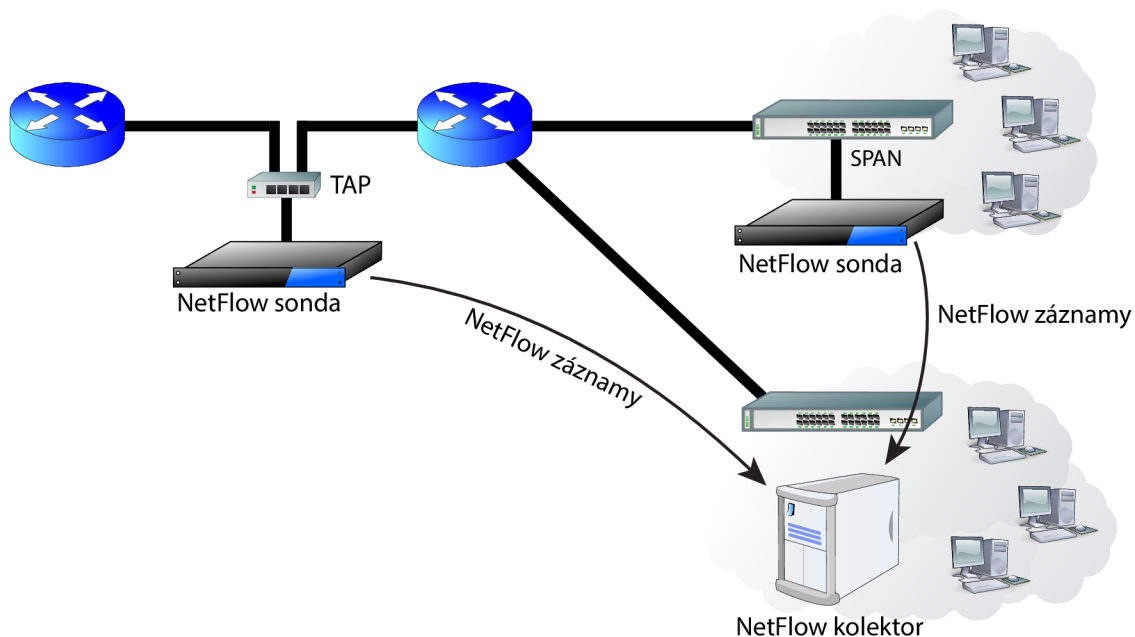
Obrázek 2.2: Architektura NetFlow využívající pasivní sondy
