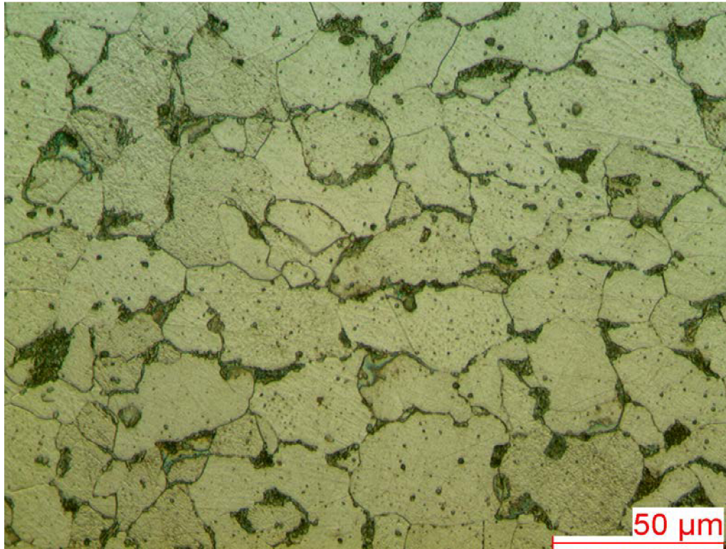
Obr. IV.15 Detail základního materiálu napříč směru tváření – převážně feritická struktura
