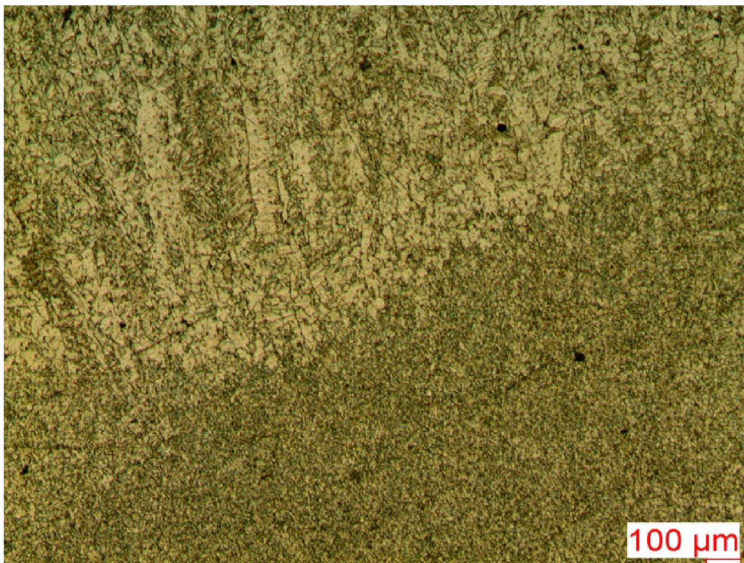
Obr. IV.20 Svarový kov – lokálně zhrublé zrna postupným pokládáním materiálu
