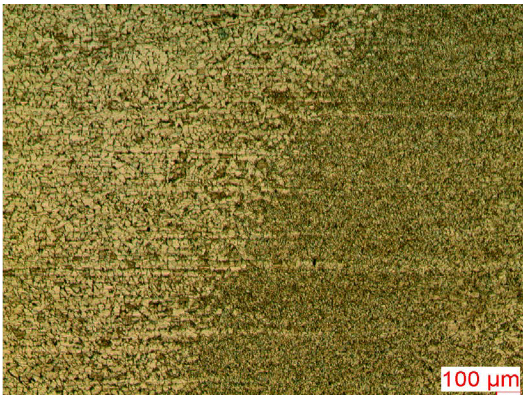
Obr. IV.18 Přejímová vrstva tvářený materiál/svar – struktura je plynule promíšena
