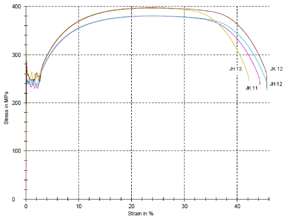
Obr. I.2 Tahové křivky základního tvářeného materiálu svaru plech/odlitek
