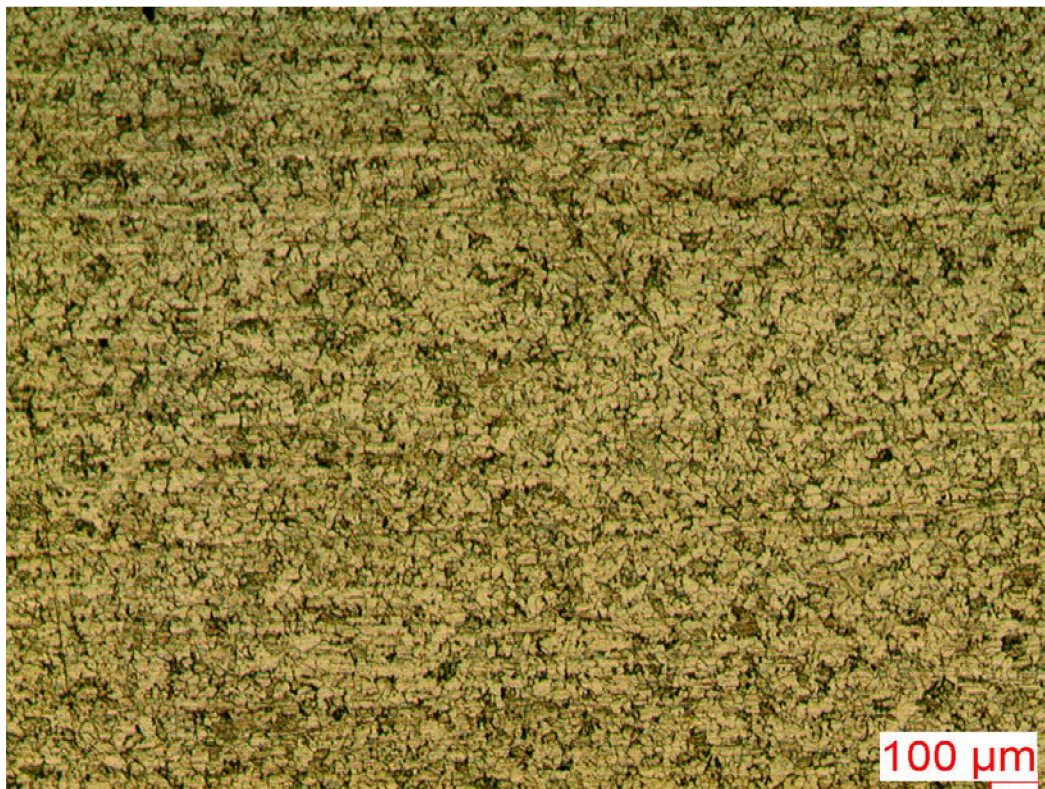
Obr. IV.12 Základní tvářený materiál ve směru válcování – řádkovitá feritická struktura
