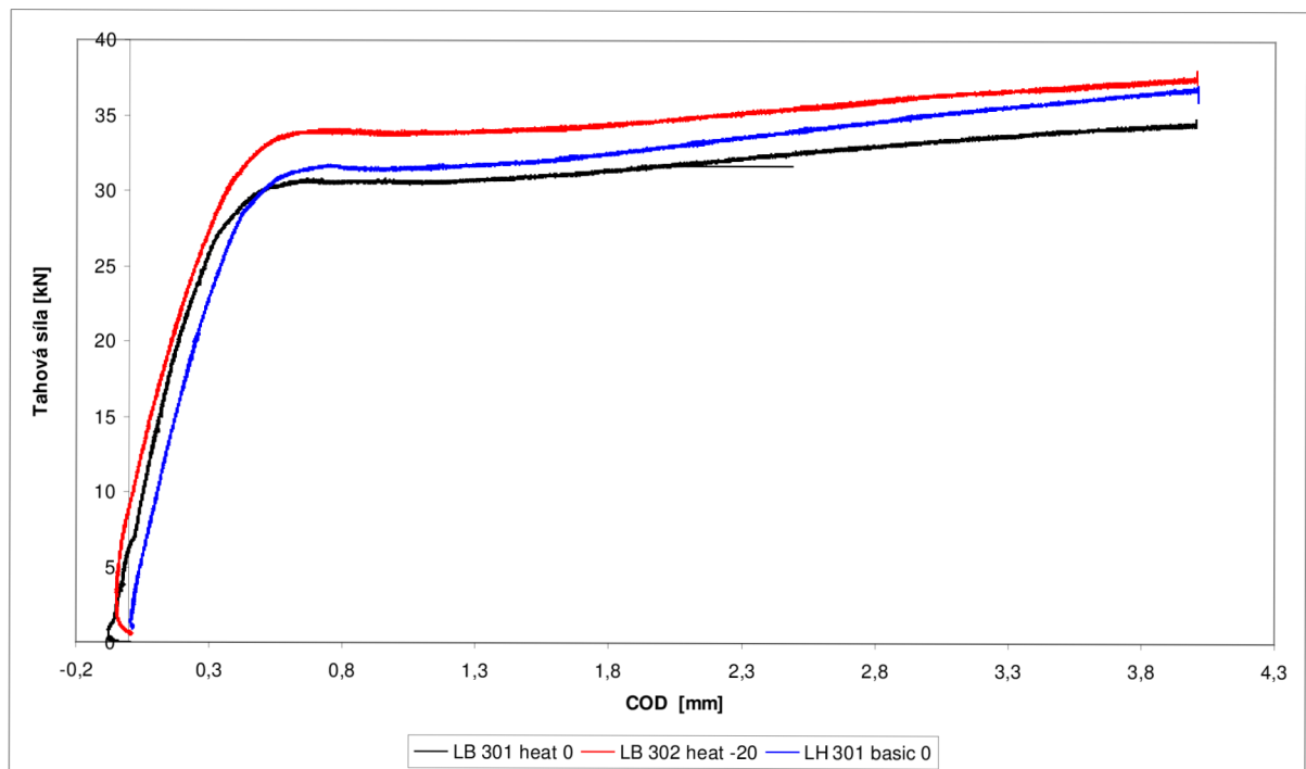
Obr. II.1 Zatěžovací křivky zkoušky lomové houževnatosti. LB 301- tepelně ovlivněná zóna, T = 0^{\circ}\text{C} ; LB 302 - tepelně ovlivněná zóna, T = -20^{\circ}\text{C} ; LH 301 -základní materiál, T = 0^{\circ}\text{C} .
