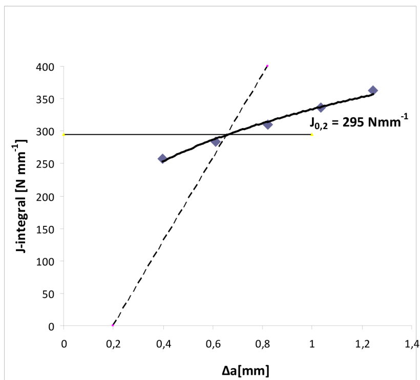
Obr. 15c J - \Delta a křivka zkušebního tělesa LH 303
