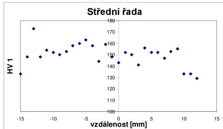
Obr. 17b Průběh mikrotvrdosti HV 1 střední řady vtisků
