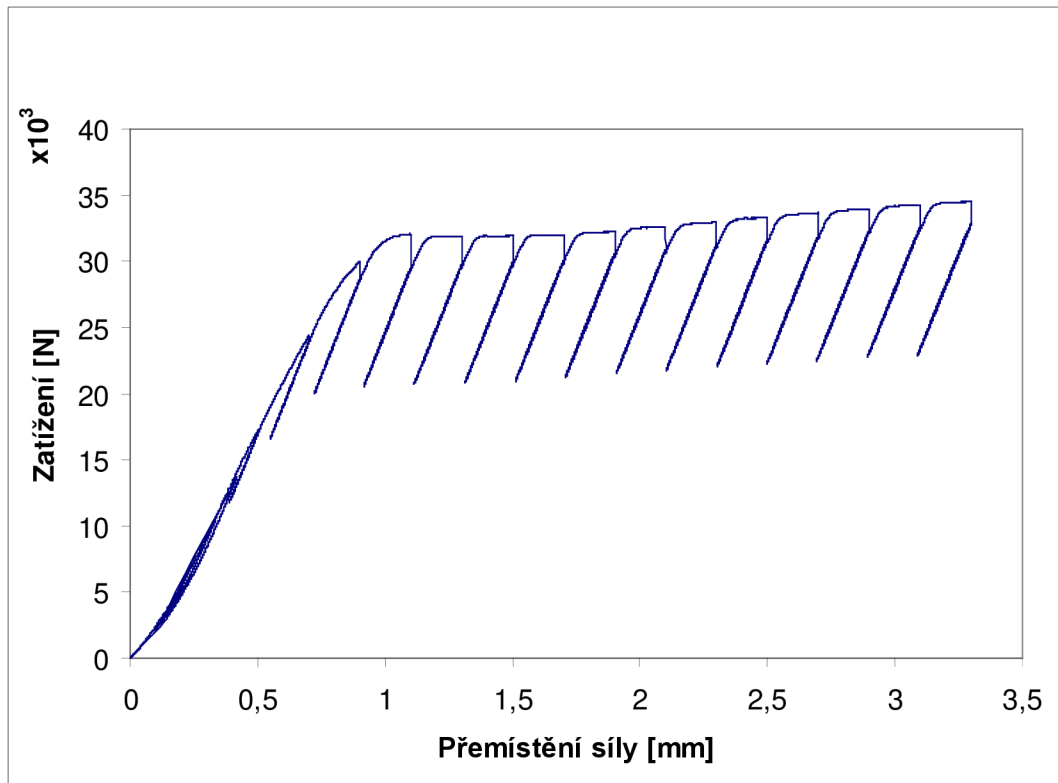
Obr. III.5 Zatěžovací křivka pro zkušební těleso LB 201
