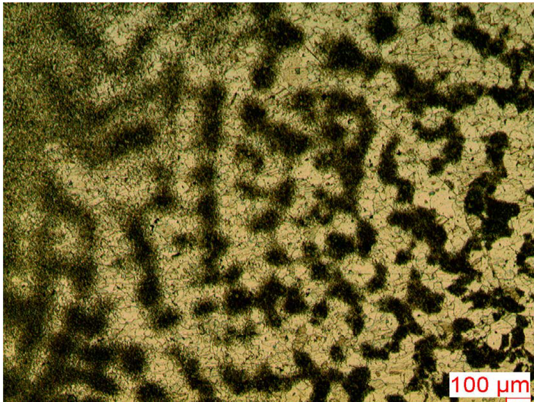
Obr. IV.19 Přechodová vrstva litý materiál/svar – feriticko-perlitická struktura, feritické zrna je rozdrobeno
