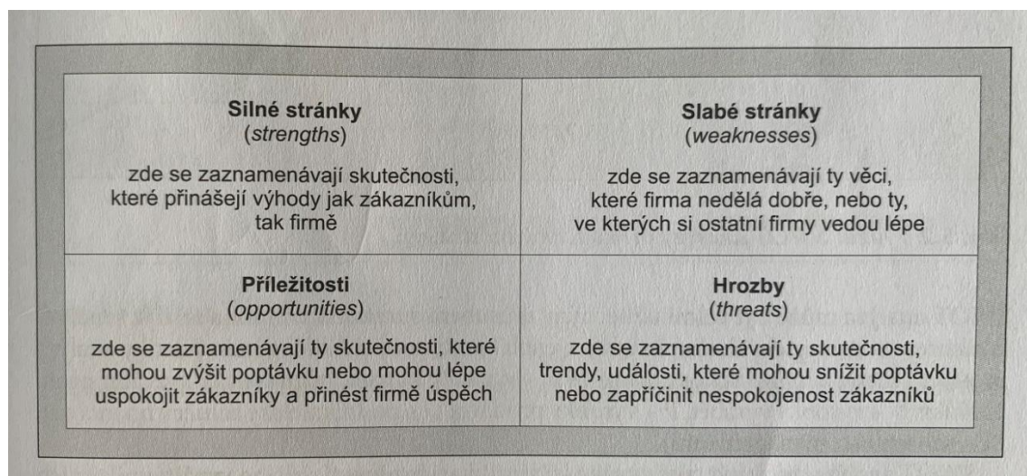
Obrázek 7: SWOT analýza
