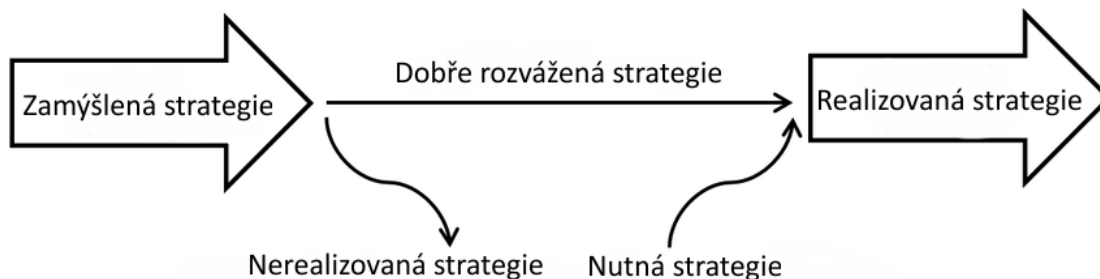
Obrázek 1: Typy strategií
