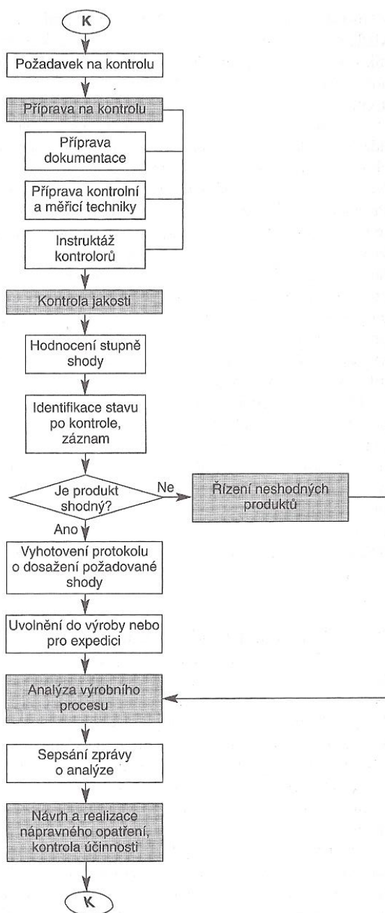
Obr. 4) Průběh procesu kontroly kvality [1]
