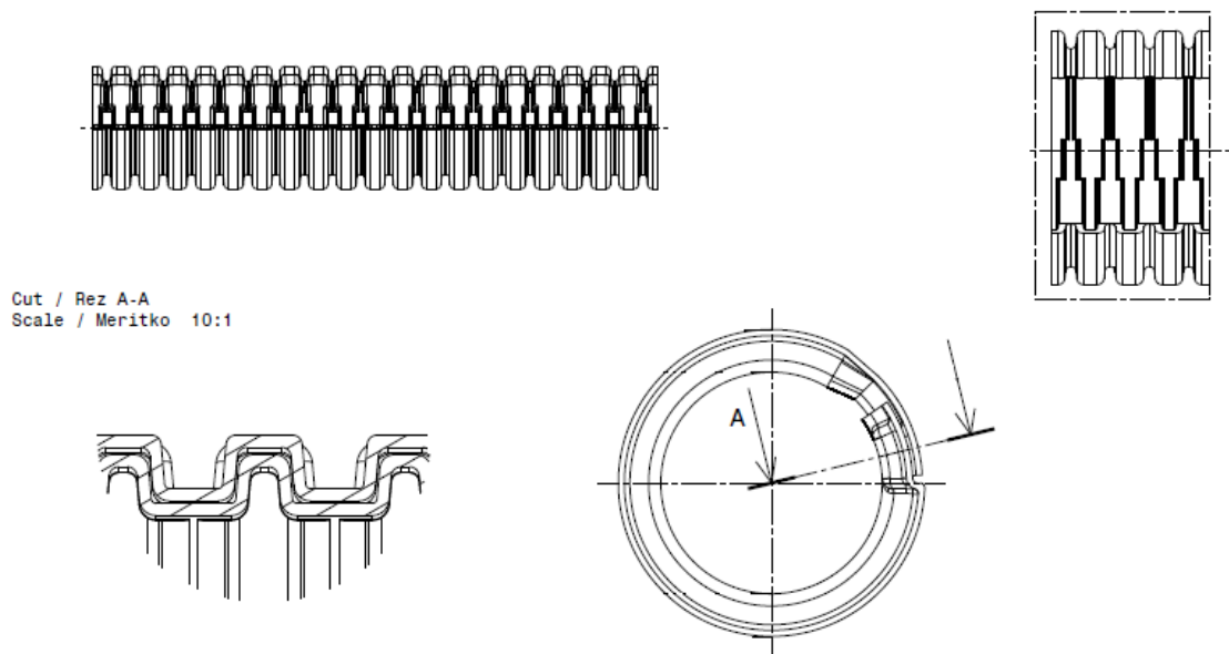
Obr. 36) Nákres dílu 461601088-03 [25]
