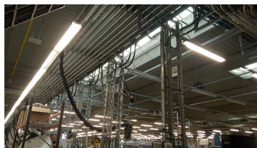
Obr. 21) Potrubí pro přenos směsí po výrobní hale [18]
