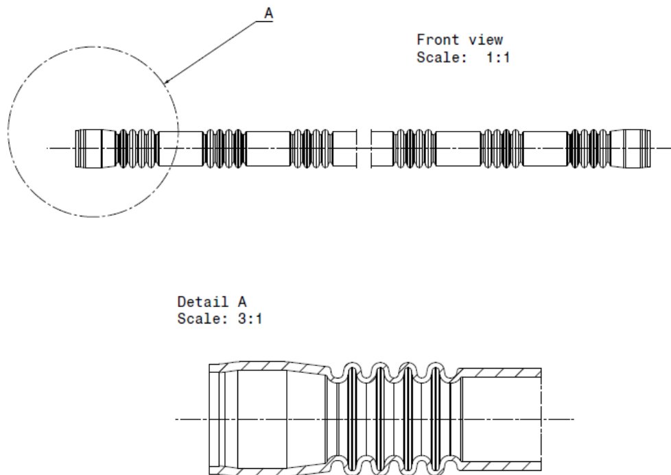
Obr. 39) Nákres dílu 36008952-03 [25]
