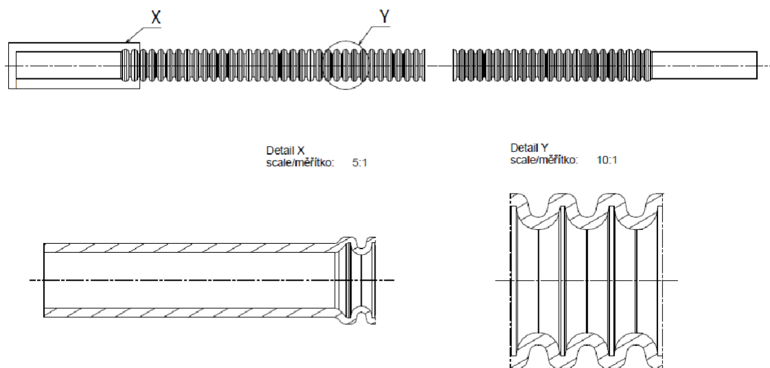
Obr. 44) Nákres dílu 36049791-03 [25]
