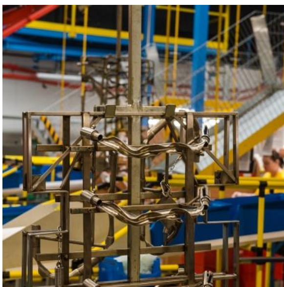
Obr. 27) Ukázka tvarovací formy [25]
