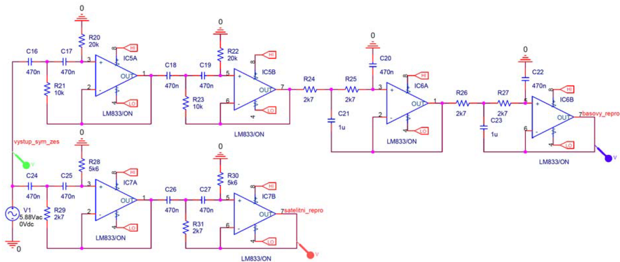
Obr. 5.2: Schéma simulované aktivní výhybky.
