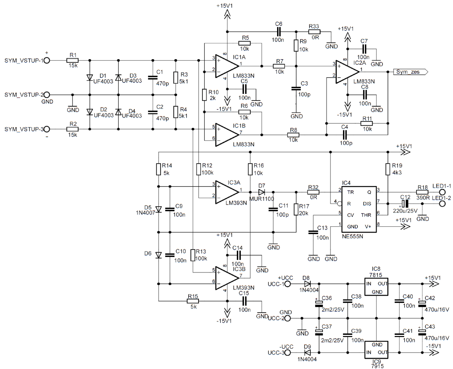
Obr. 4.1: Schéma vstupního předzesilovače.
