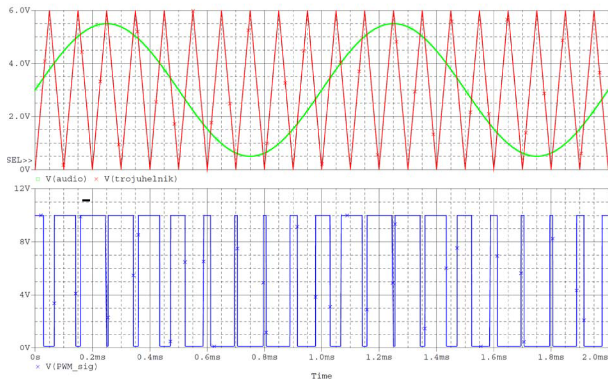
Obr. 2.3: Vstupní průběhy napětí do komparátoru a výstupní pulsně šířkově modulovaný signál.
