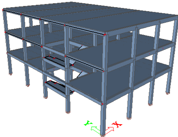
Obr. 1 – 3D model konstrukce I
