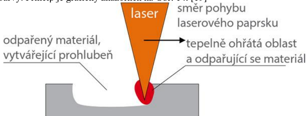
Obr. 14 - Hlubkové gravírování [20]
