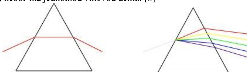
Obr. 7 Monochromatismus
