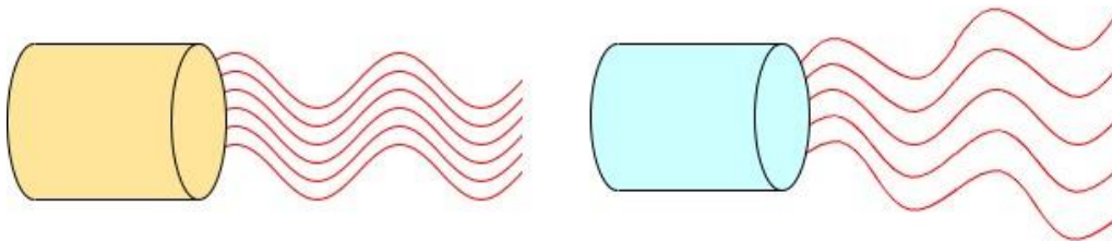
Obr. 9 - Směrovost
