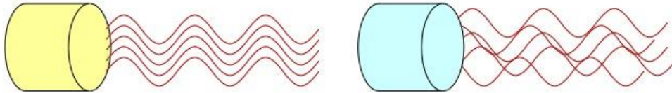
Obr. 8 – Koherentnost
