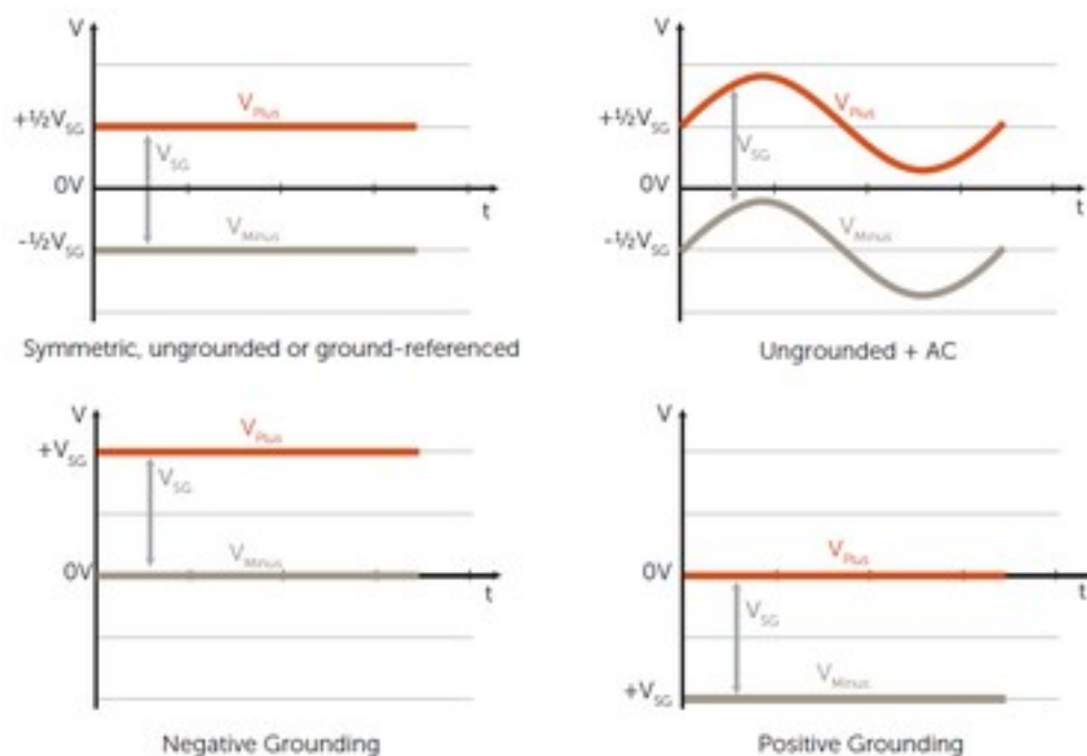
Obrázek 18 - Napěťový potenciál závisí na systému uzemnění, což může mít tyto čtyři základní klasifikace.[15]
