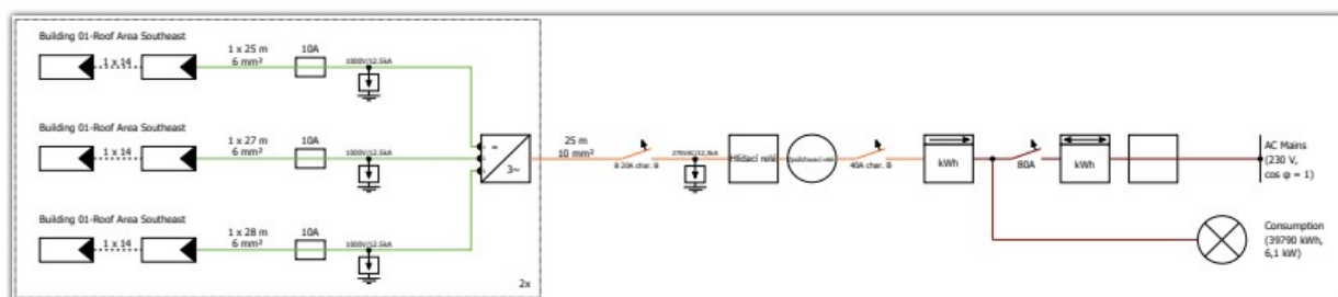
Obrázek 30 – Schéma FVE
