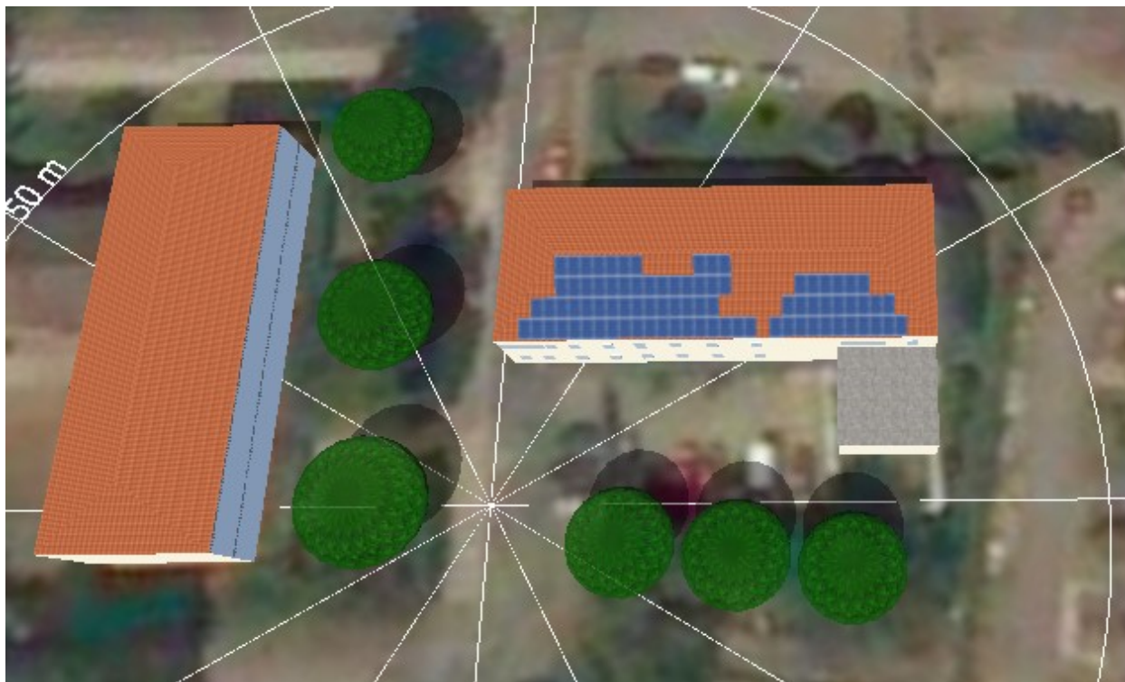
Obrázek 27 – Objekty, které se podepisují na stínění FVE
