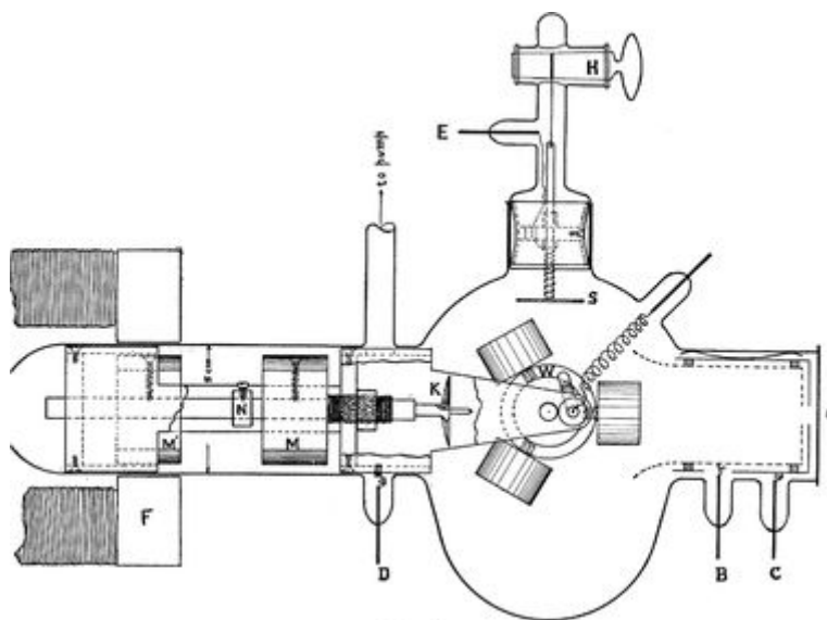
Obrázek 5- Experimentální zařízení prof. Millikana "dílna ve vakuu" [6]
