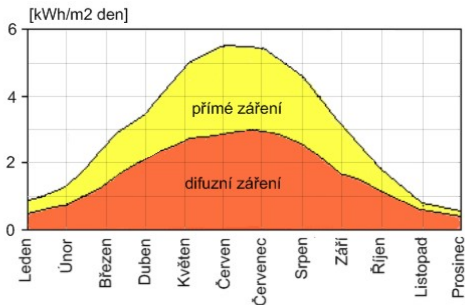
Obrázek 2- Přímé vs difuzní záření[2]
