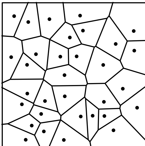
Obrázek 2.10: Voroného diagram
