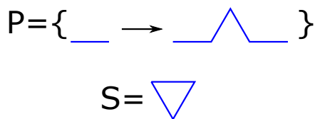
Obrázek 2.12: Systém G_{koch}
