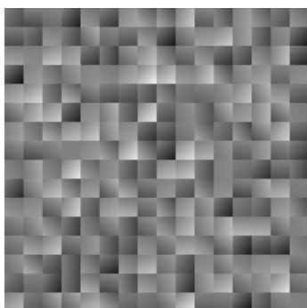
Obrázek 2.5 Gradientní šum
