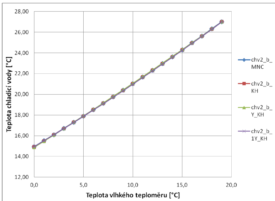
Graf 3: Vykreslení modelů pro parametry F_{chv}=67000t/h a Q=950MW věž 1B
