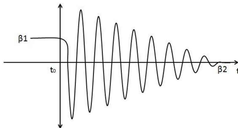
Obrázek 13 Kývání synchronního stroje
