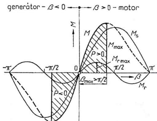
Obrázek 8 Moment synchronního stroje s vyjádřenými póly [11]
