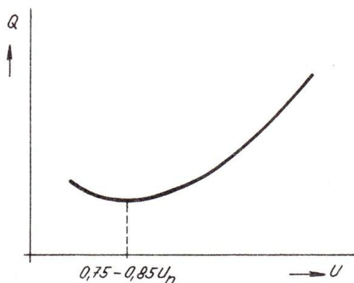
Obrázek 20 Závislost jalového výkonu spotřebičů na napětí[13]
