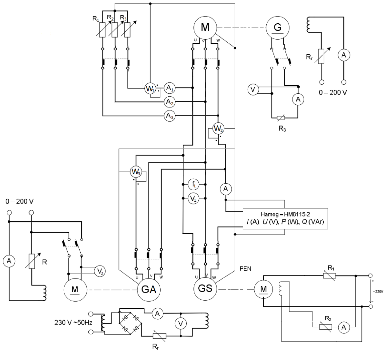
Obrázek 24 Schéma zapojení zkušební ostrovní sítě
