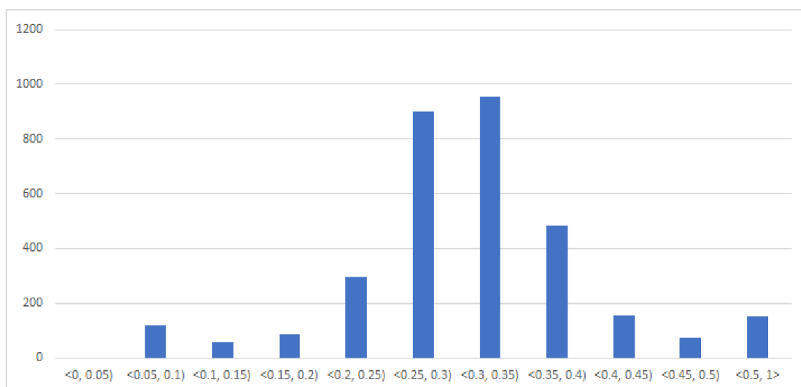
Obrázok 7.19. Graf znázorňujúci ohodnotenie morfovaného odtlačku voči pôvodným. Predstavuje početnosť ohodnotení (vertikálna os) voči odpovedajúcim odtlačkom v intervaloch po 0,5 nadobudnutého skóre verifikácie (horizontálna os). V prípade porovnania dvoch rovnakých odtlačkov nadobudnuté skóre sa pohybuje od 0,65 vyššie. Výsledky boli získané z pôvodnej metódy morfovania bez zásahov rozšírení.
