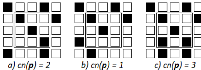
Obrázok 3.6. Typy markantov detekovateľných pomocou crossing number . [6]
