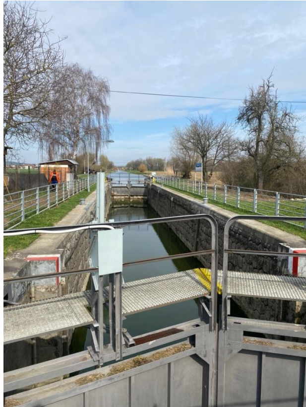
Obrázok 15 Plavebná komora Babice na Baťovom kanáli (zdroj; autor 2024).
