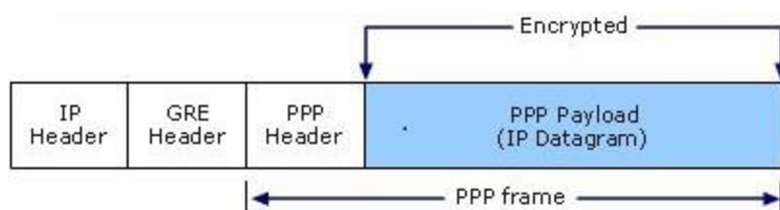
Obr. 1.5: Zapouzdření PPTP paketů
