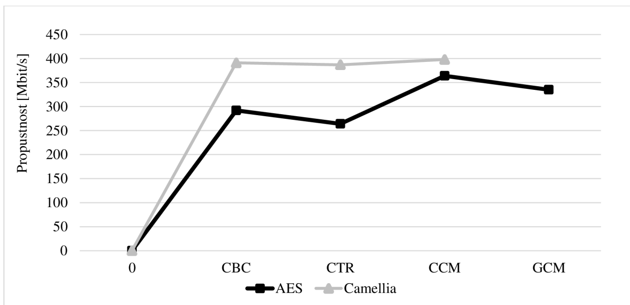
Obr. 5.2: Rychlost (download) se zapouzdřením ESP (AES a Camellia)
