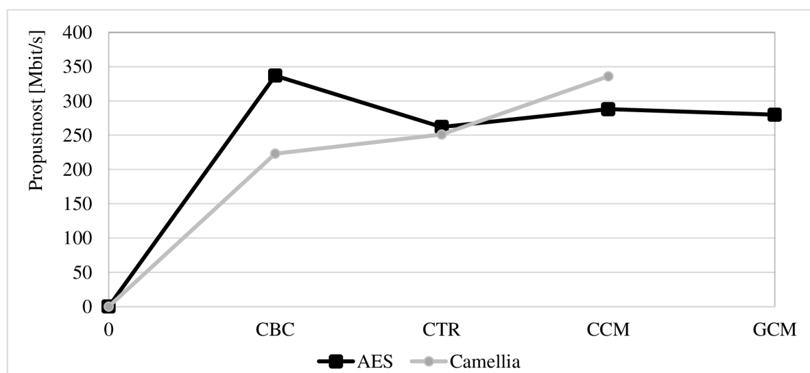
Obr. 5.1: Rychlost (download) při metodách šifrování IKE (AES a Camellia)
