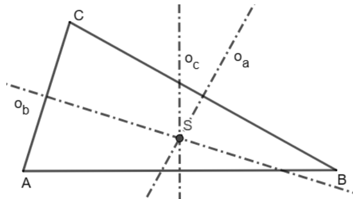
Obr. č. 24 Důkaz průsečíku os stran trojúhelníku ABC
