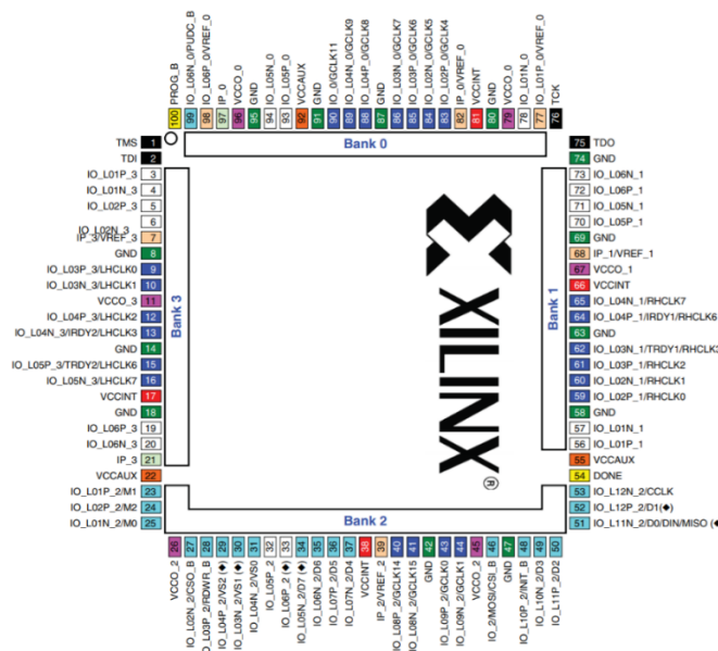
Obrázek 8 – Označení a využití vývodů kontroléru XC3S50A [21]
