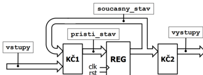
Obrázek 5 – Blokové schéma Moorova stavového automat [19]
