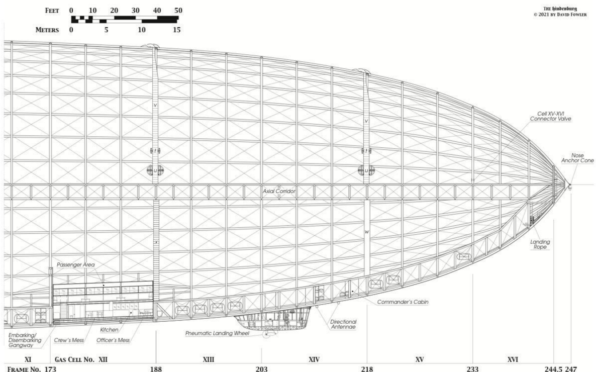
Obr. 2-6 Výkres přídí Hindenburgu s palubami ukrytými uvnitř kostry [25]
