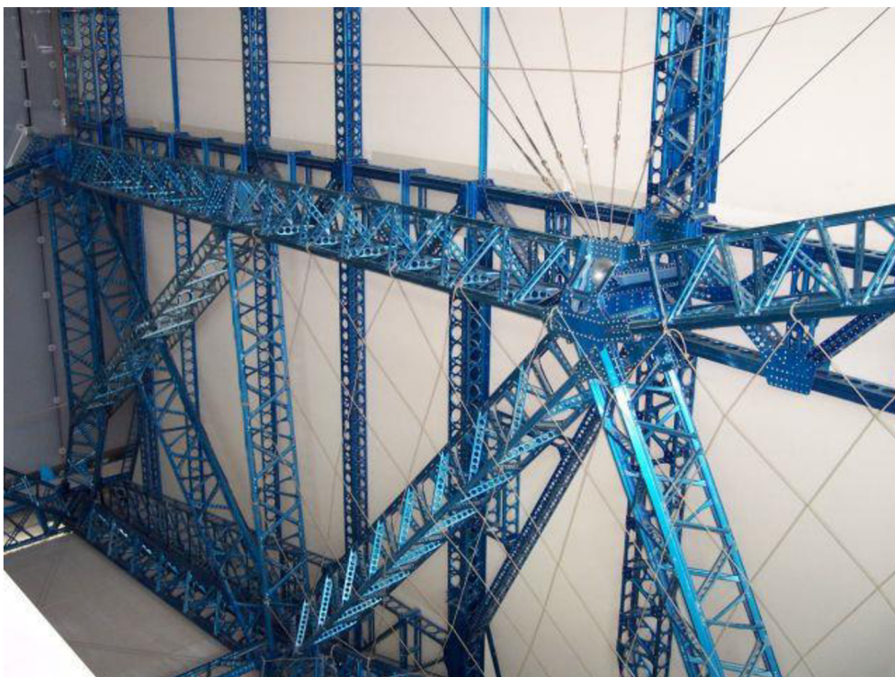
Obr. 3-14 Nýtovaná konstrukce kostry z trojúhelníkových duralových nosníků [27]
