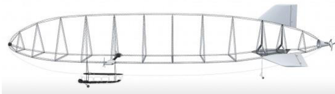
Obr. 6-1 Konstrukce Zeppelinu NT [6]
