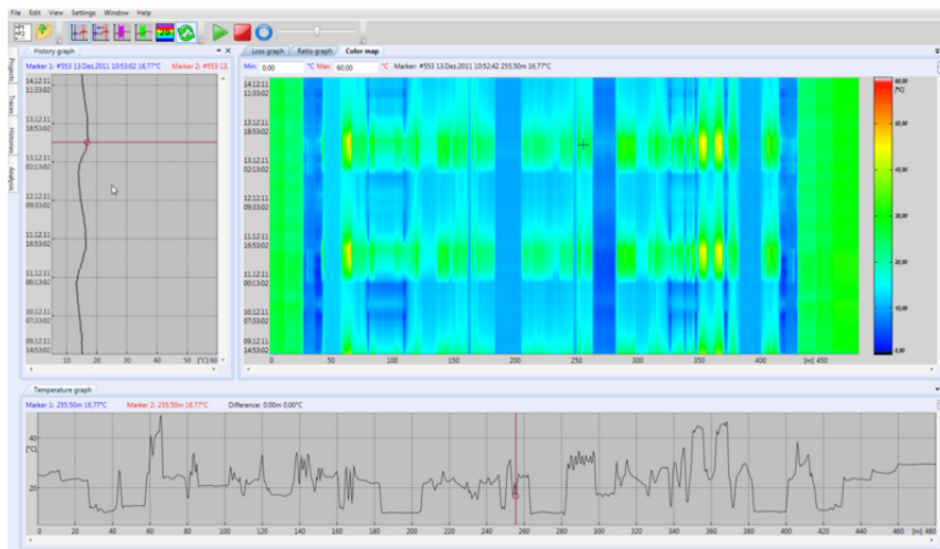
Obr. 5.6: SmartVision™ software – příklad zobrazení
