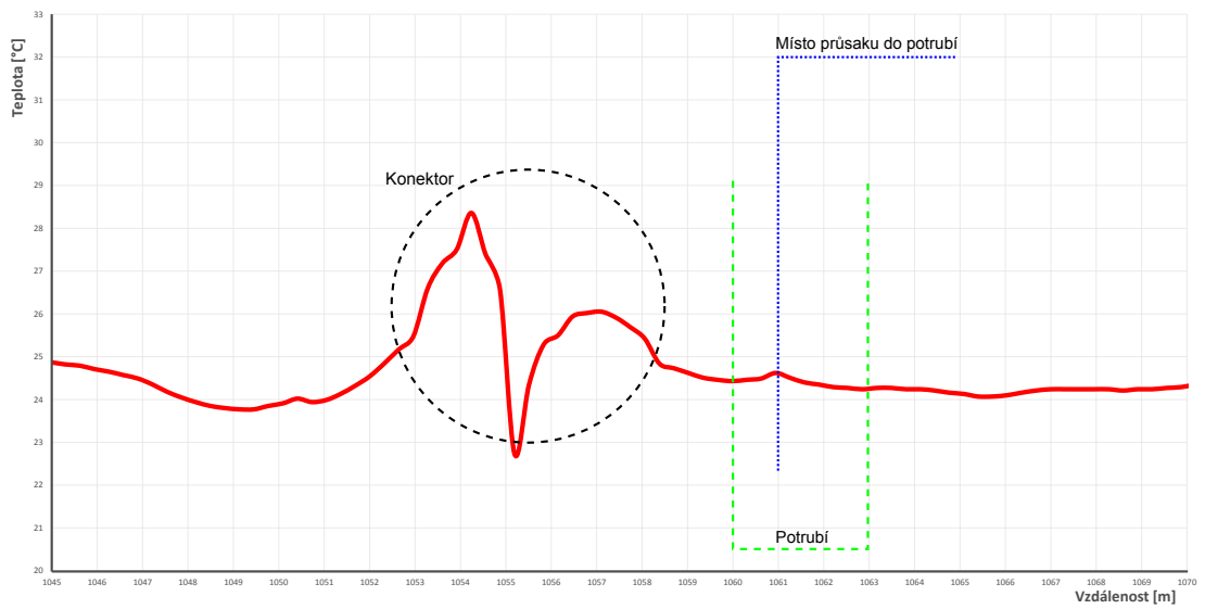
Obr. 7.8: Graf teploty – 12. minuta
