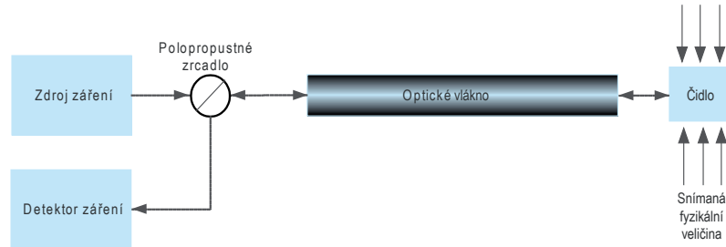
Obr. 2.3: Blokové schéma zapojení extrinžitní metody měření
